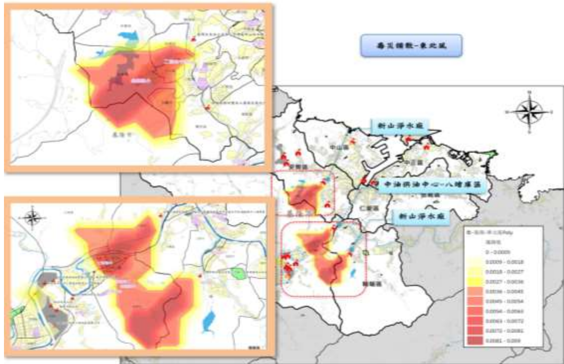
圖 65 基隆市毒災擴散風險潛勢圖(東北風)
