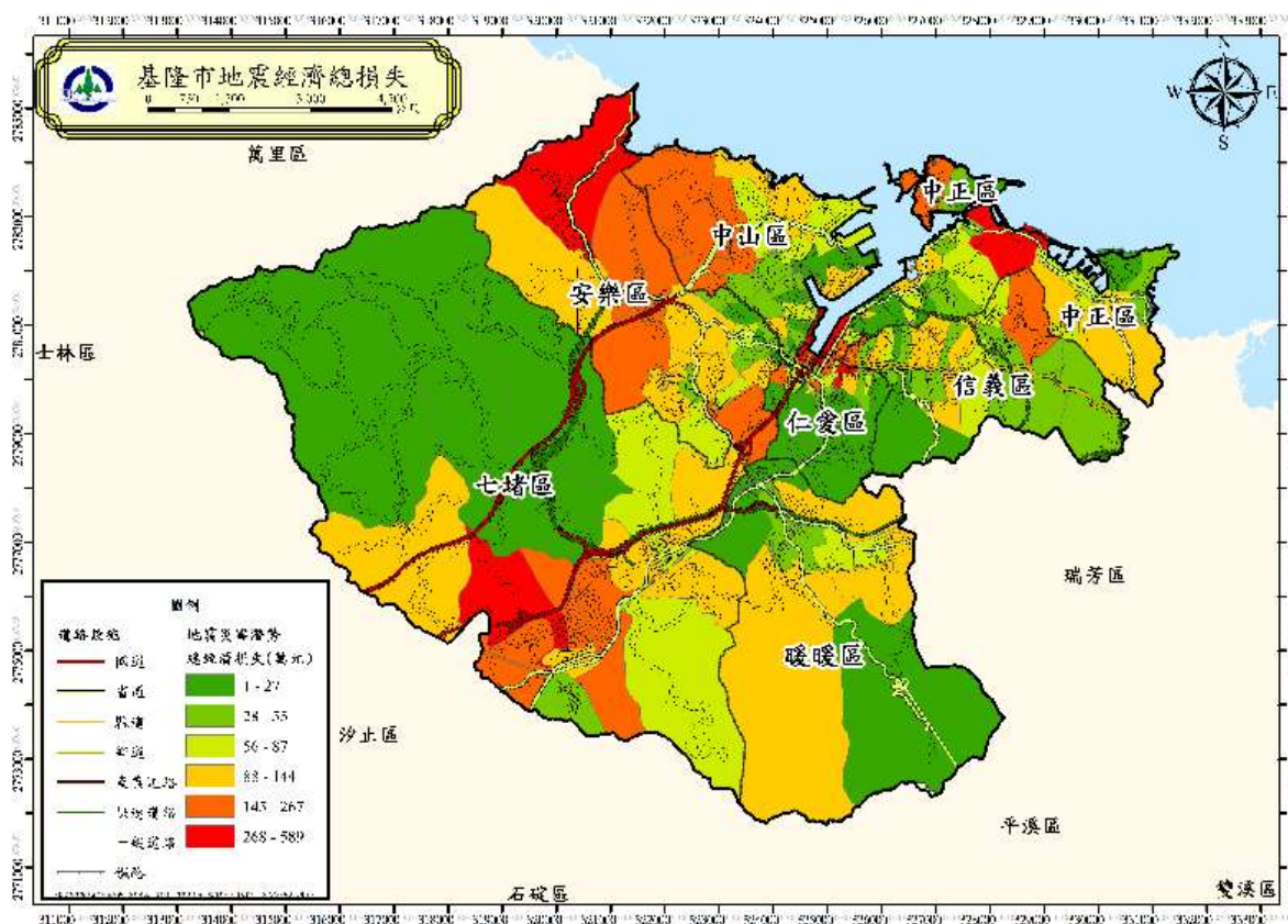
圖 37 基隆市模擬地震總經濟損失分布圖(芮氏規模 7.1)
