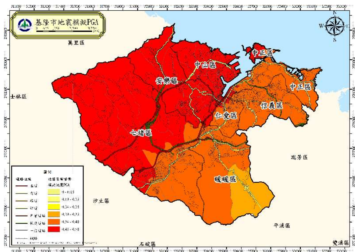
圖 38 基隆市模擬地震 PGA 分布圖(芮氏規模 7.3)
