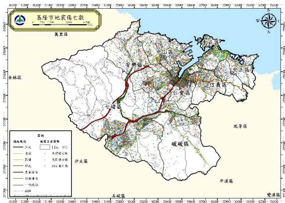
圖 39 基隆市模擬地震傷亡數(日間、夜間、假日)分布圖(芮氏規模 7.3)
