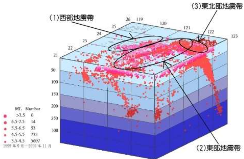
圖 26 臺灣主要三個地震帶圖
