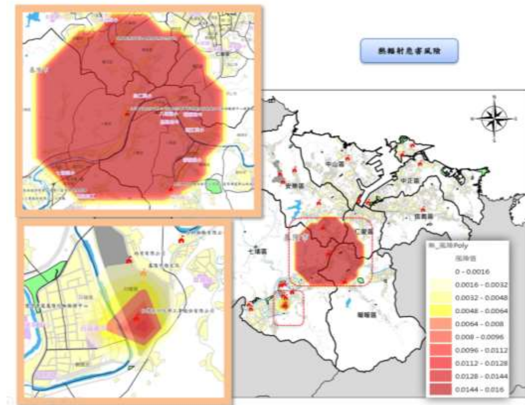
圖 61 基隆市熱輻射危害風險潛勢圖
