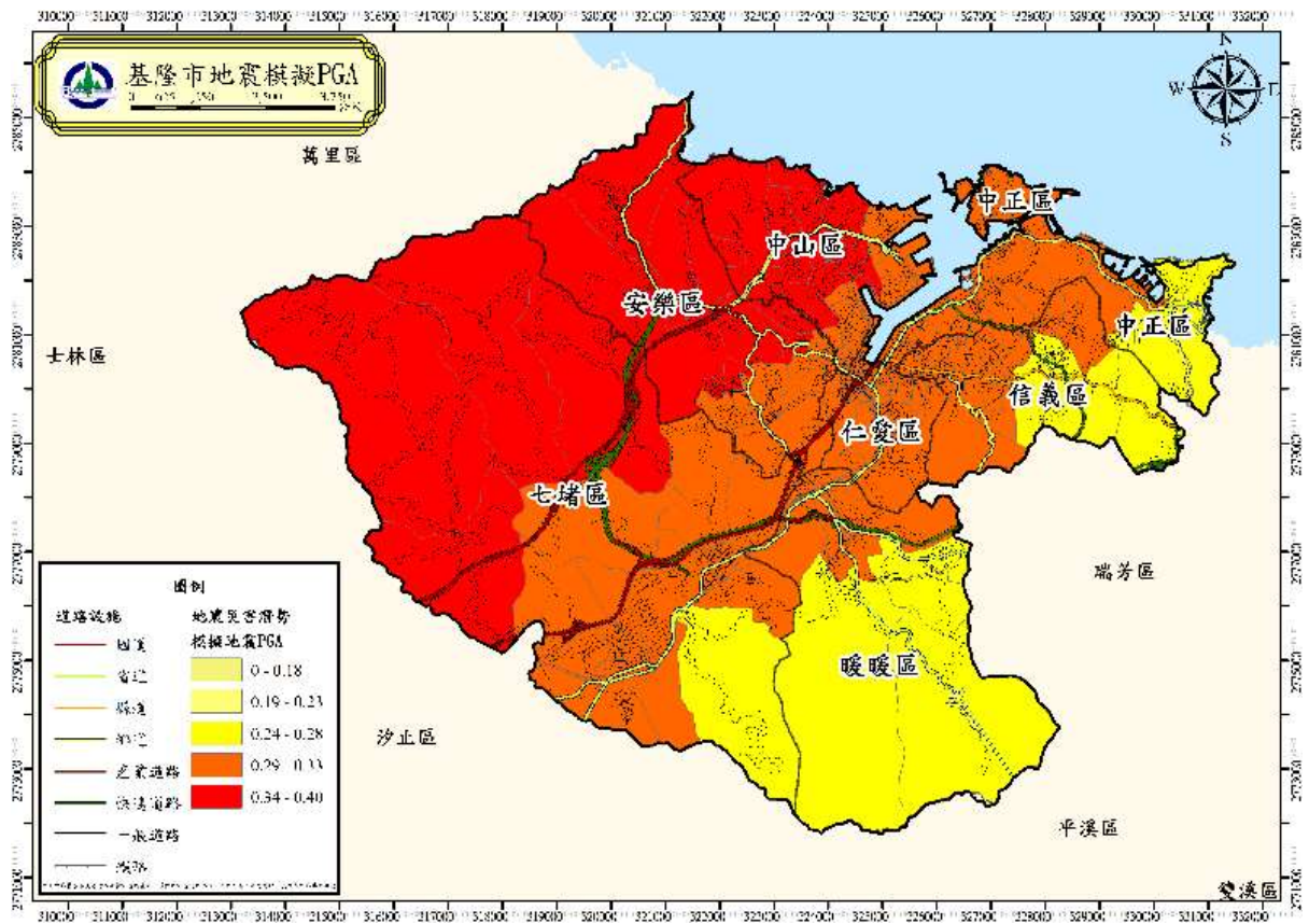
圖 28 基隆市模擬地震 PGA 分布圖(芮氏規模 6.9)
