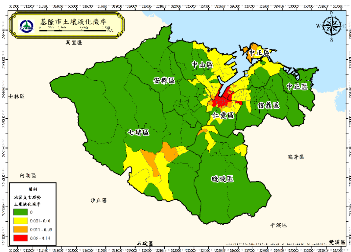
圖 31 基隆市模擬地震土壤液化機率分布圖(芮氏規模 6.9)
