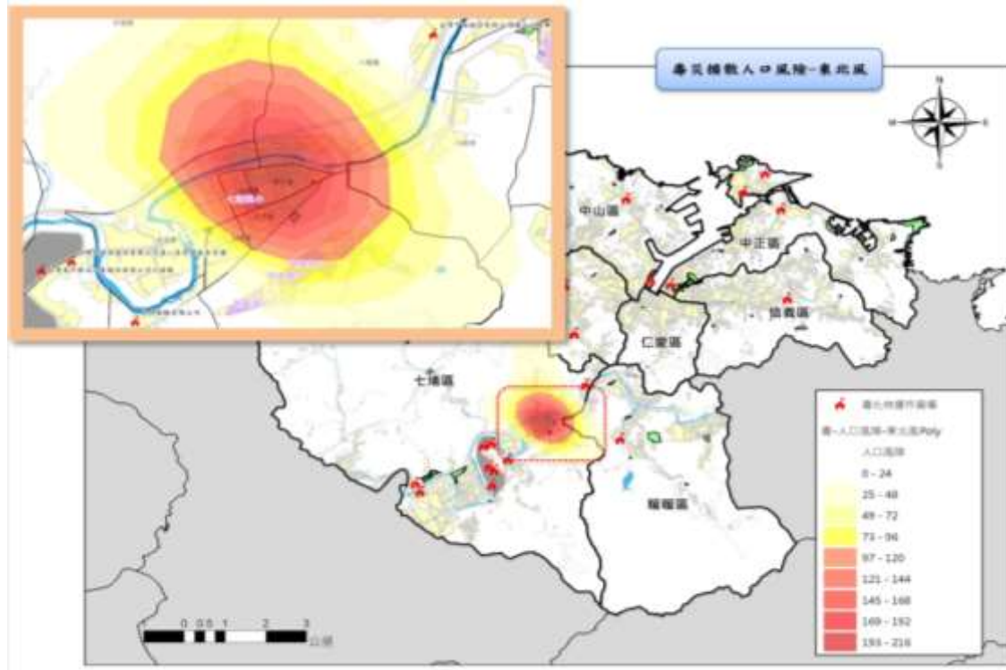
圖 66 基隆市毒災擴散人口風險潛勢圖(東北風)
