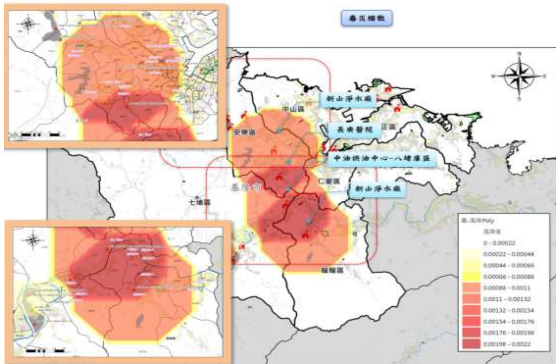
圖 63 基隆市毒性擴散危害風險潛勢圖(無風向)
