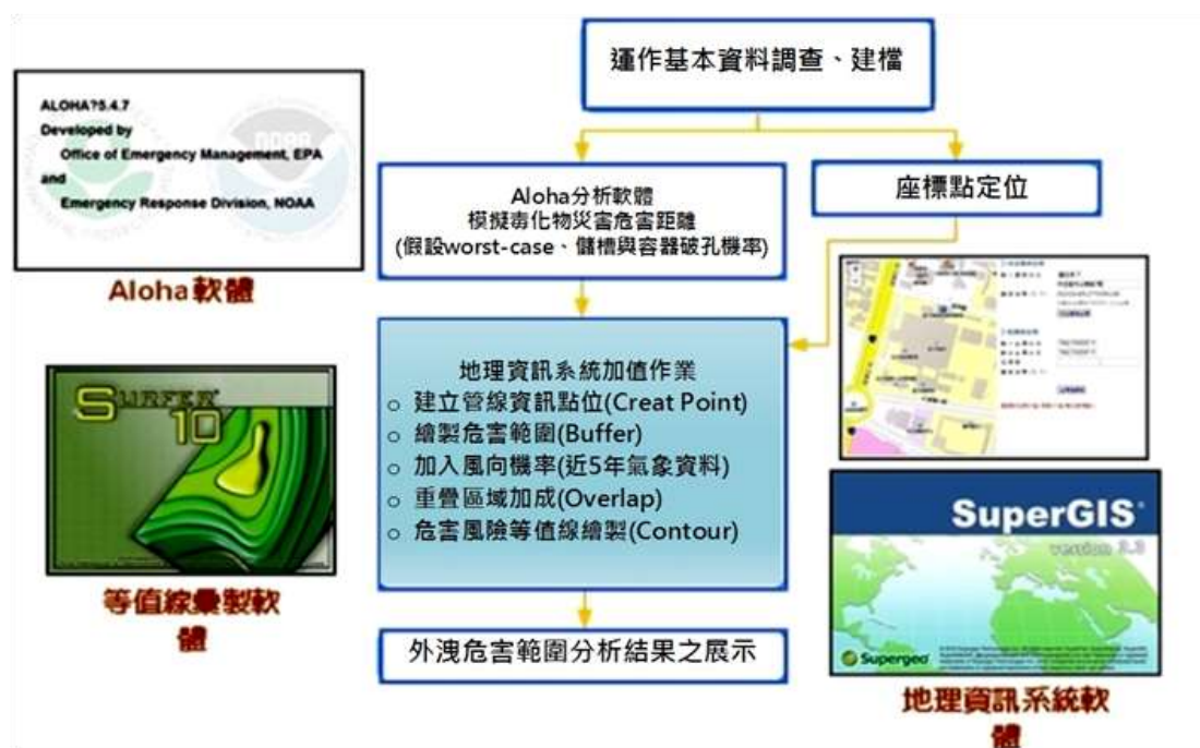
圖 53 毒災風險評估方法流程
