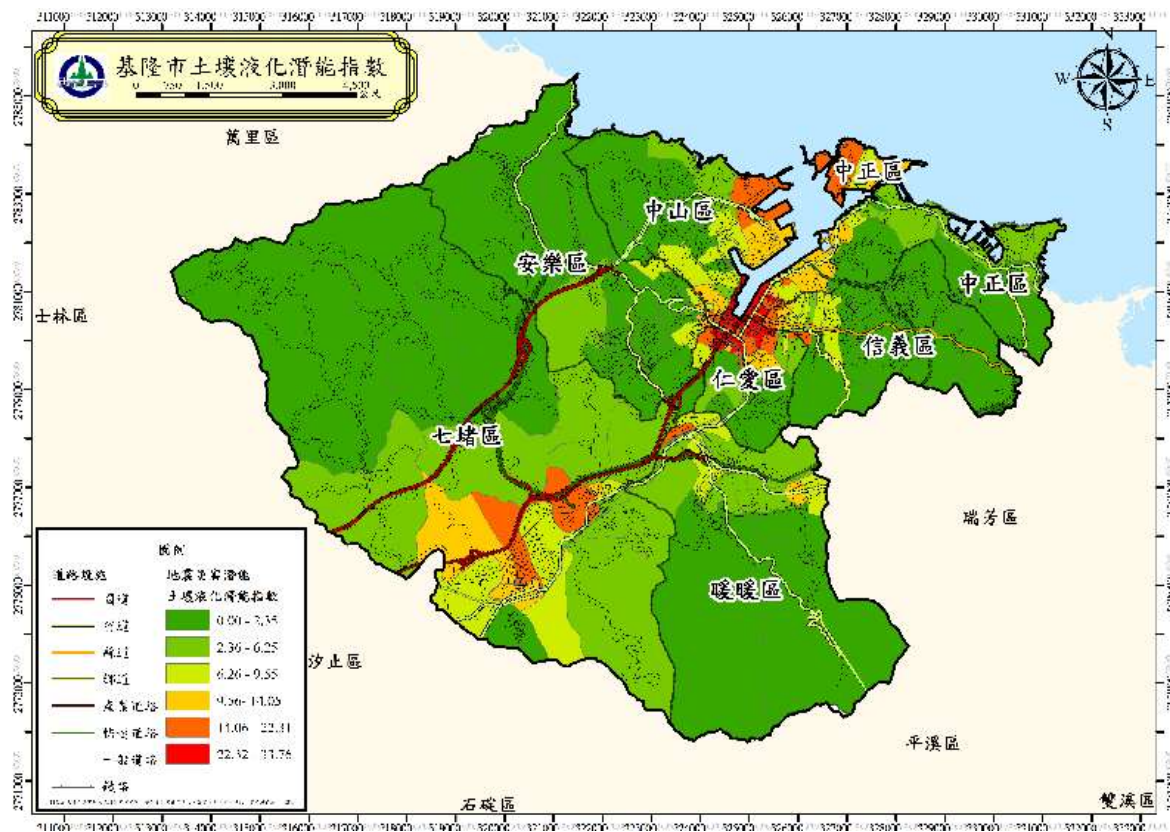
圖 35 基隆市模擬地震建物損害分布圖(芮氏規模 7.1)
