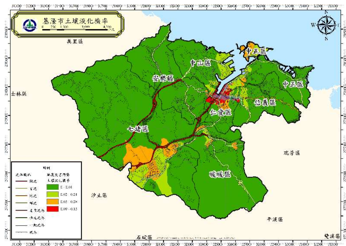
圖 41 基隆市模擬地震土壤液化機率分布圖(芮氏規模 7.3)
