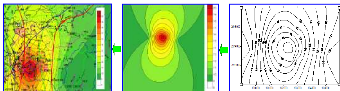
圖 57 風險等值線繪製與圖層套疊
