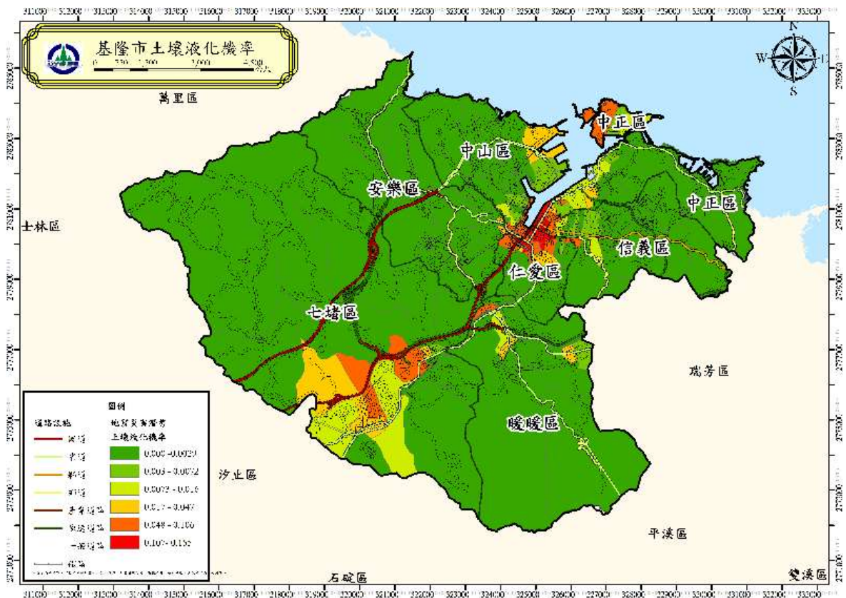
圖 36 基隆市模擬地震土壤液化機率分布圖(芮氏規模 7.1)
