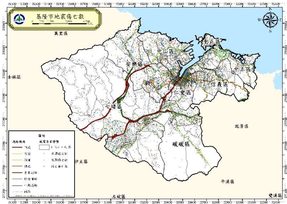
圖 29 基隆市模擬地震傷亡數(日間、夜間、假日)分布圖(芮氏規模 6.9)
