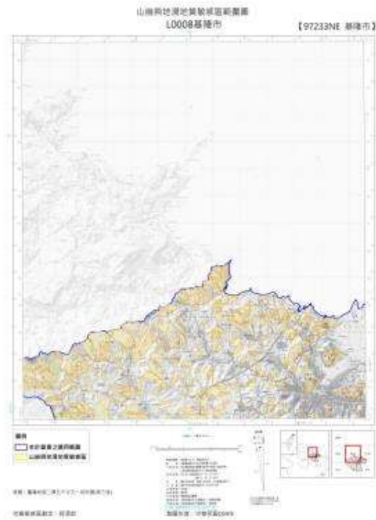
圖 22 基隆市山崩與地滑地質敏感區範圍圖 97233NE 基隆市
