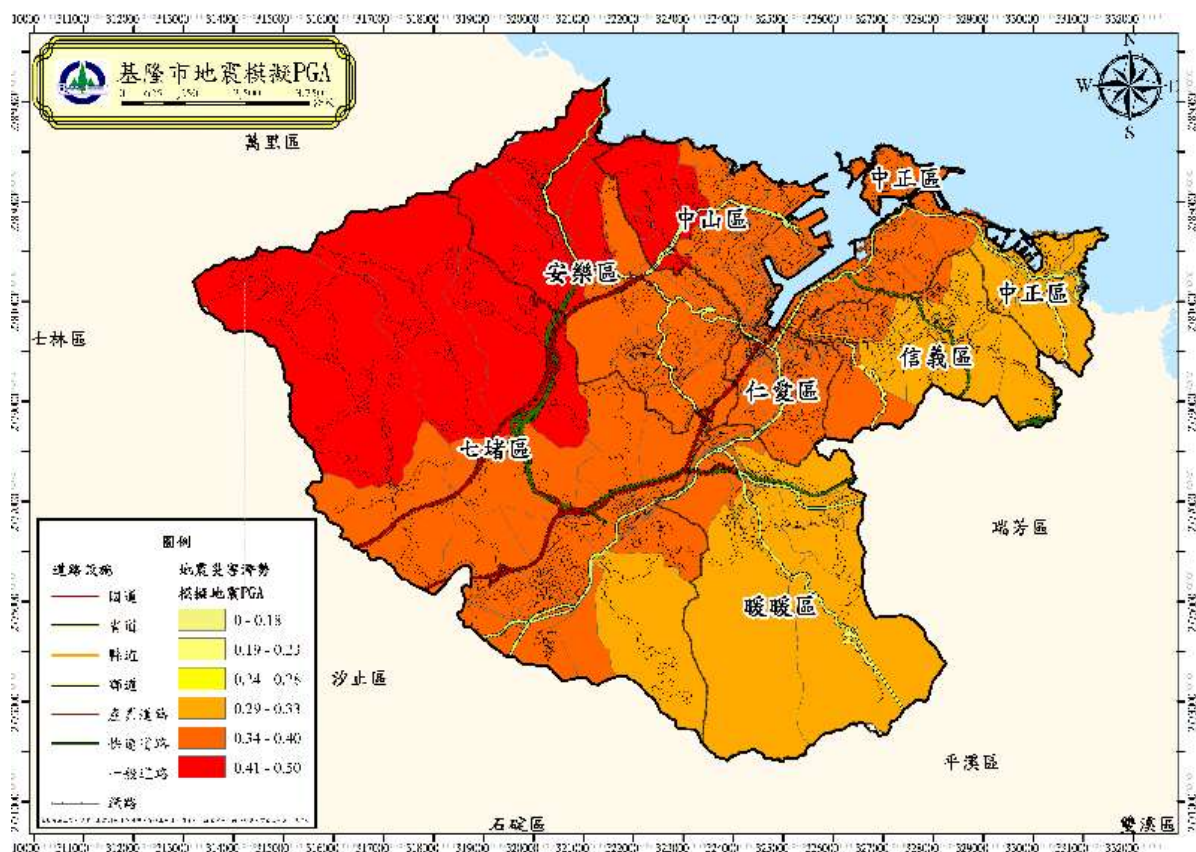
圖 33 基隆市模擬地震 PGA 分布圖(芮氏規模 7.1)
