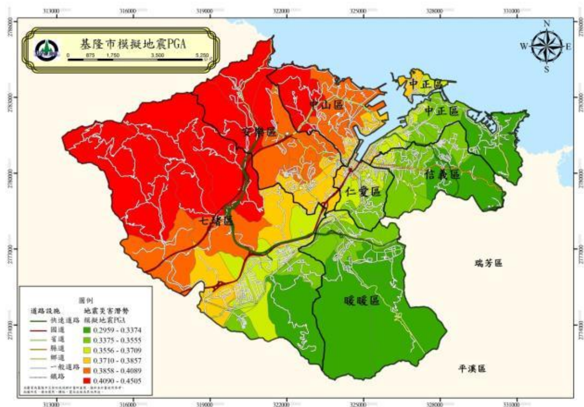
圖 30 基隆市模擬地震 PGA 分布圖(芮氏規模 7.1)
