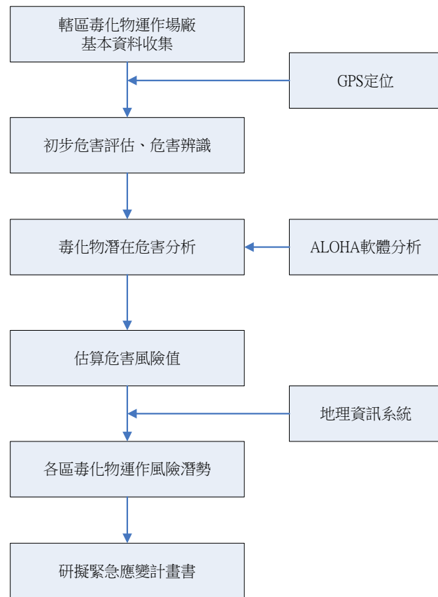
圖 50 毒性化學物質運作場廠風險評估架構
