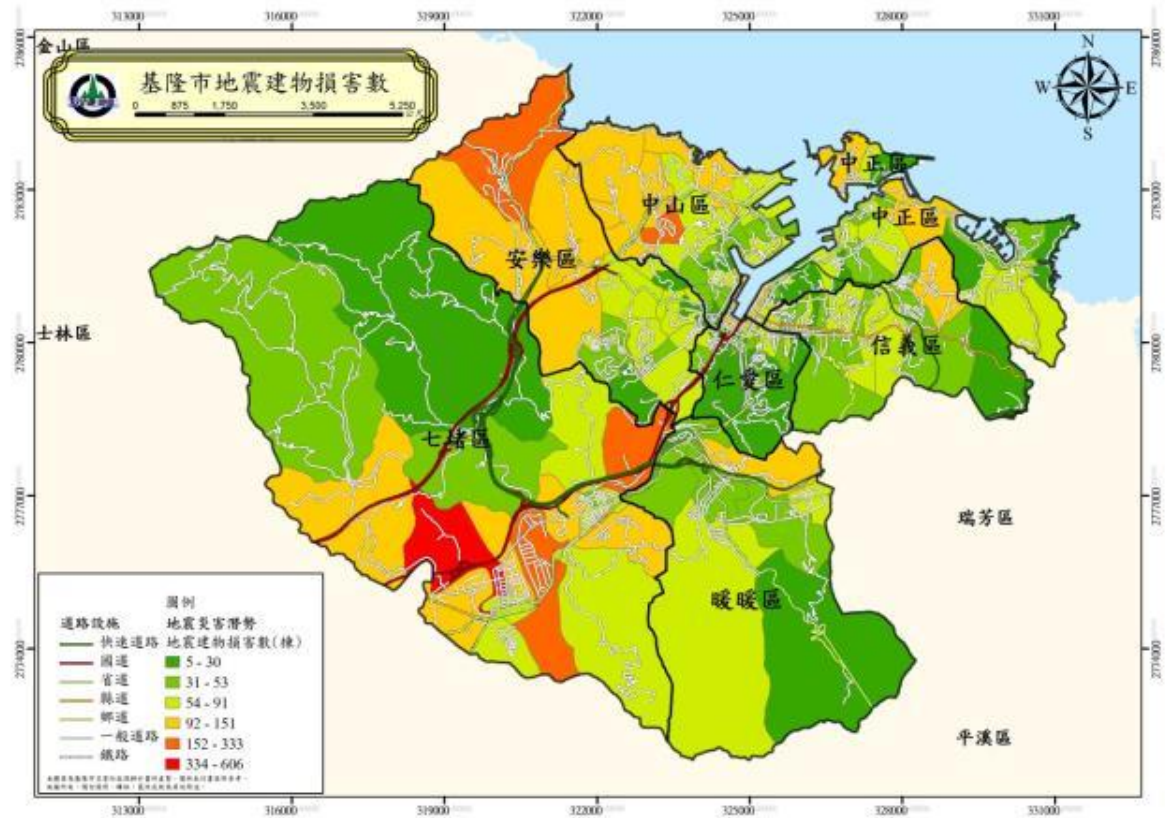
圖 27 基隆市模擬地震建物損害分布圖(芮氏規模 6.9)
