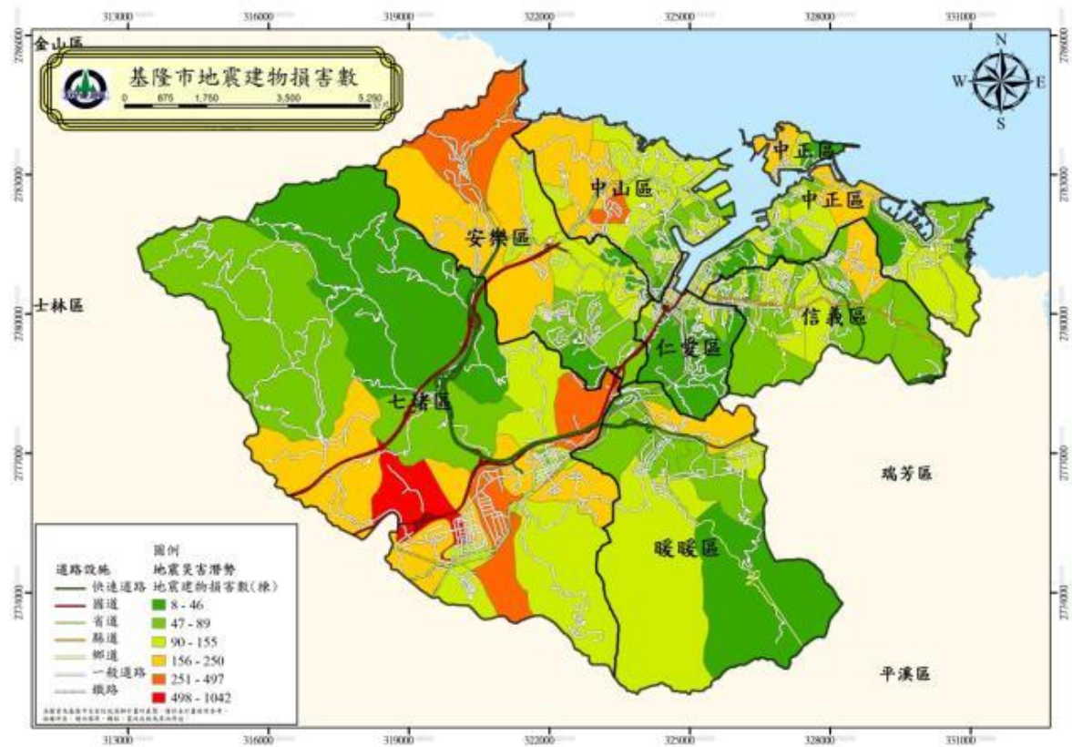
圖 37 基隆市模擬地震建物損害分布圖(芮氏規模 7.3)
