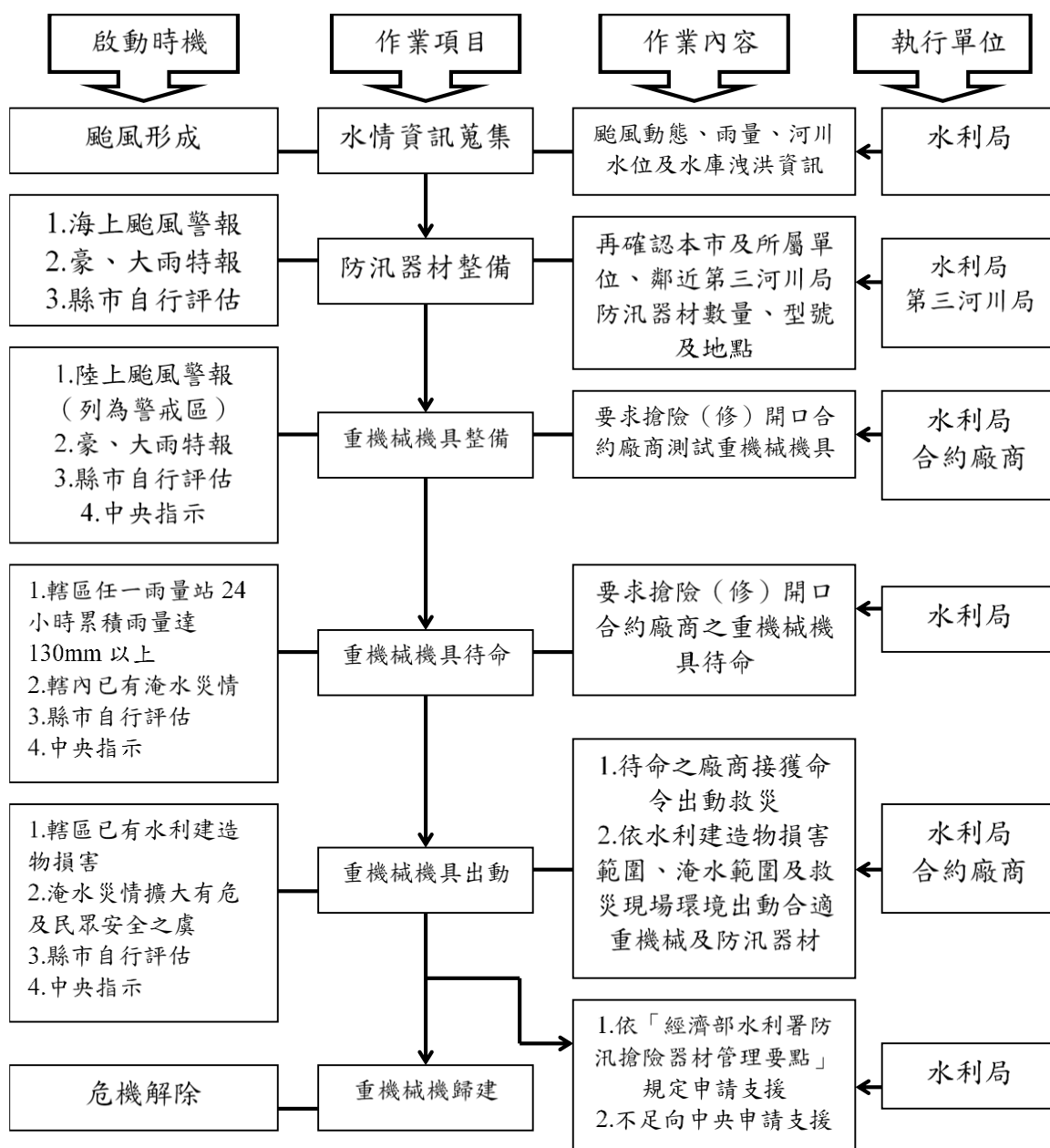
圖 16-2-2 防汛器材運用流程圖
