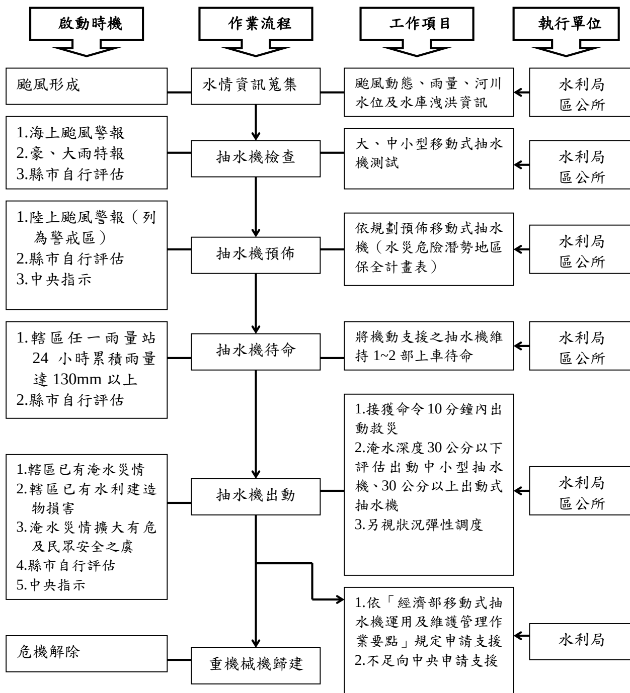
圖 16-2-3 移動式抽水機運用流程圖
