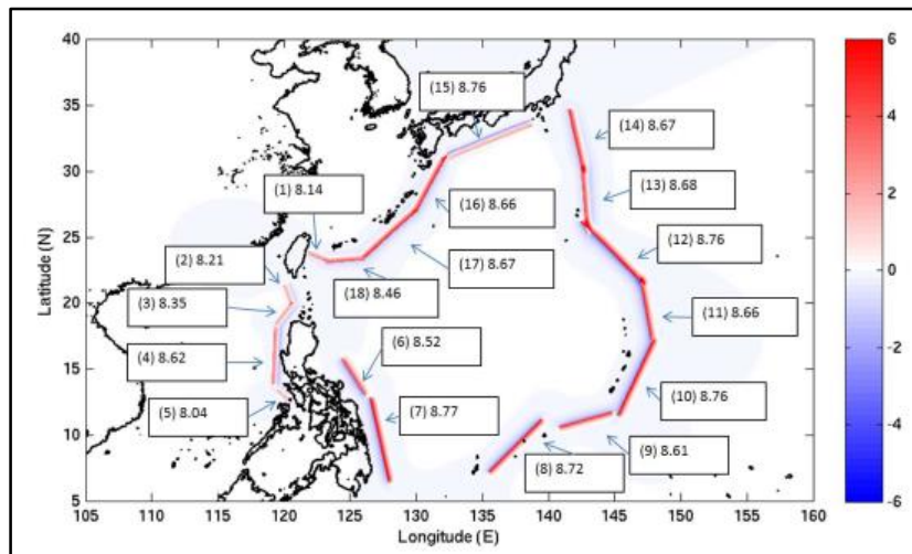
圖 5-1-2 海溝型海嘯源編號、地震矩規模與分布位置圖
