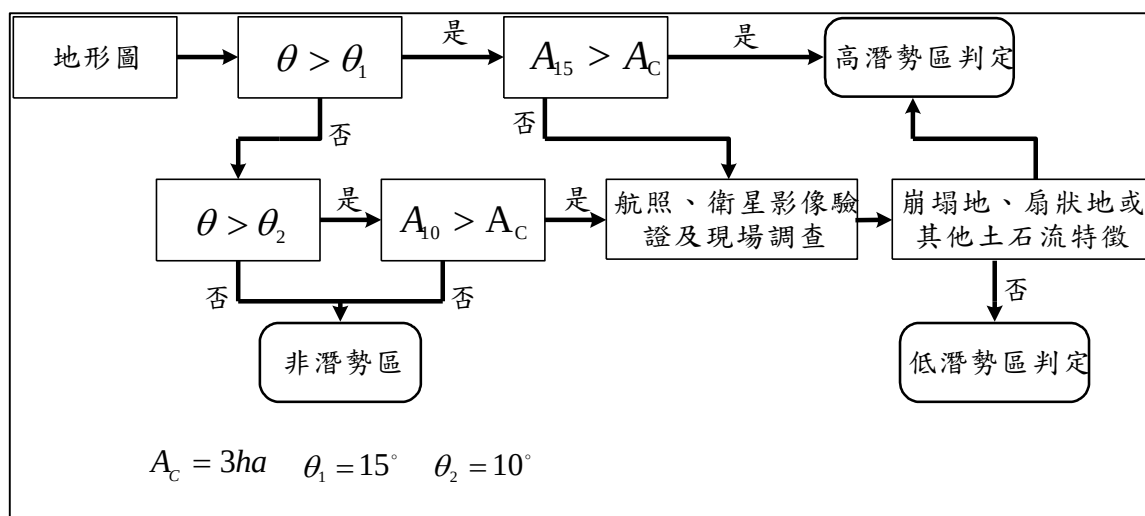
圖 3-1-16 土石流潛勢分析流程圖
