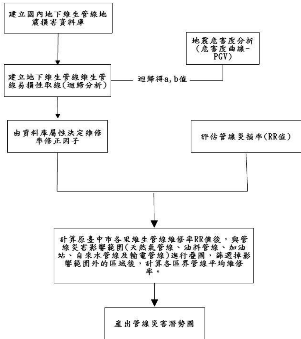
圖 10-1-5 管線地震災害評估架構
