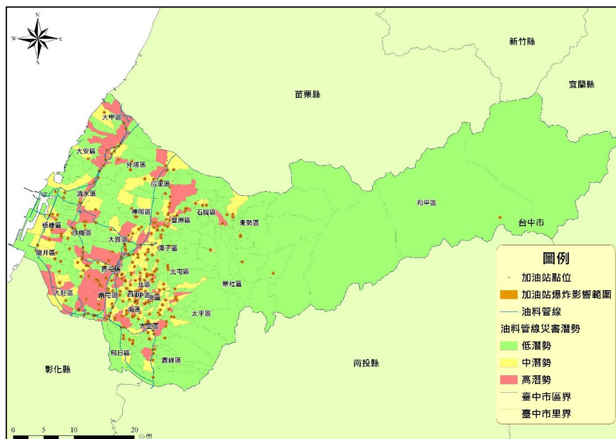
圖 10-1-6 臺中市油料管線災害潛勢圖
