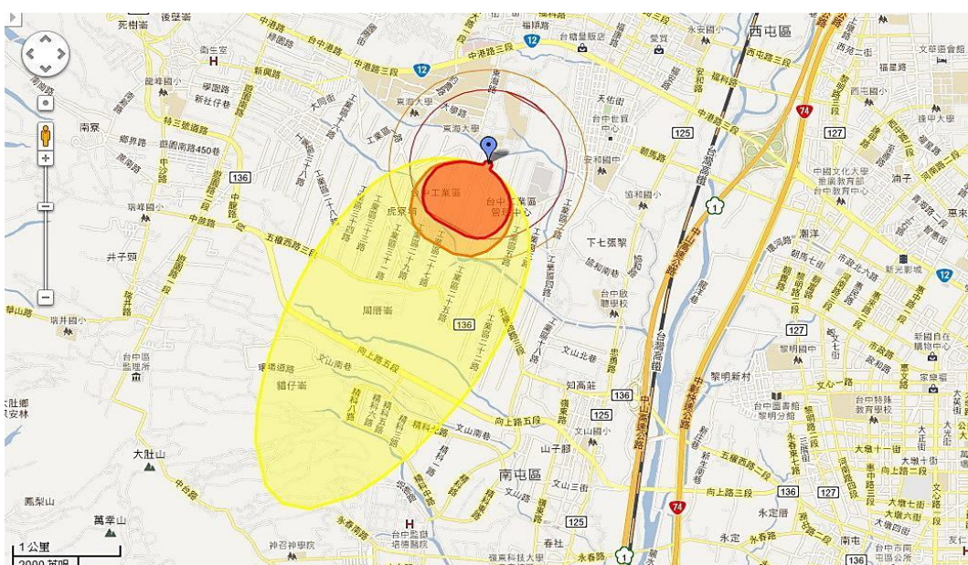
圖 6-1-3 ALOHA 程式推估結果
