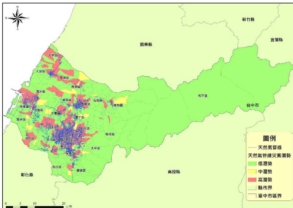
圖 10-1-9 臺中市天然氣管線災害潛勢圖
