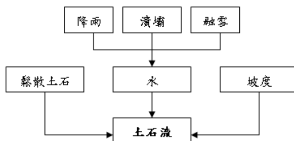
圖 4-1-1 形成土石流之基本要件示意圖
