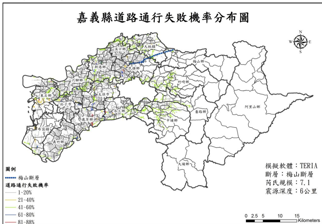
圖 3-2-11 嘉義縣道路通行失敗機率分布圖
