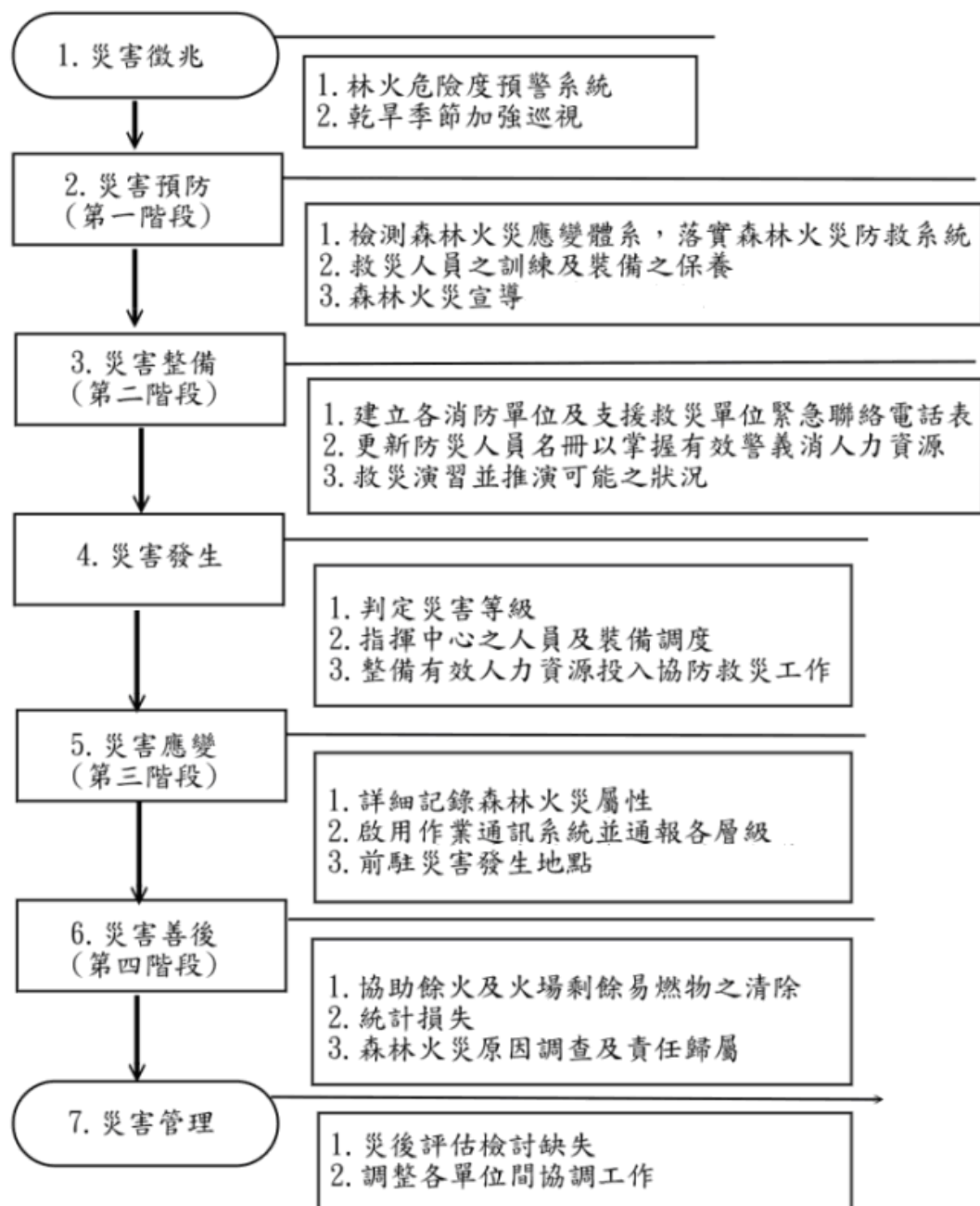
圖 6-6- 1 森林火災防救標準作業流程圖
