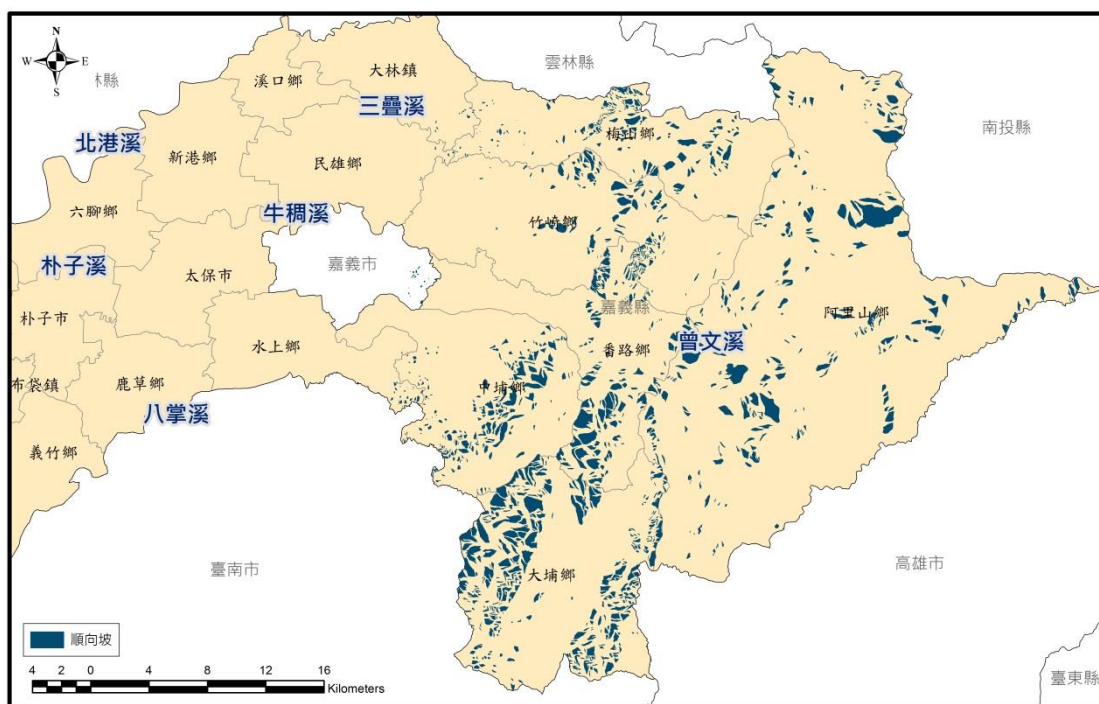
圖 4-2-2 嘉義縣順向坡位置圖
