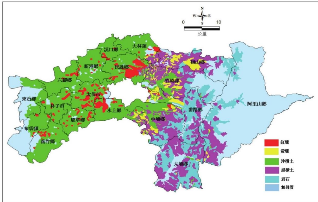
圖 1-2- 17 嘉義縣地質圖
