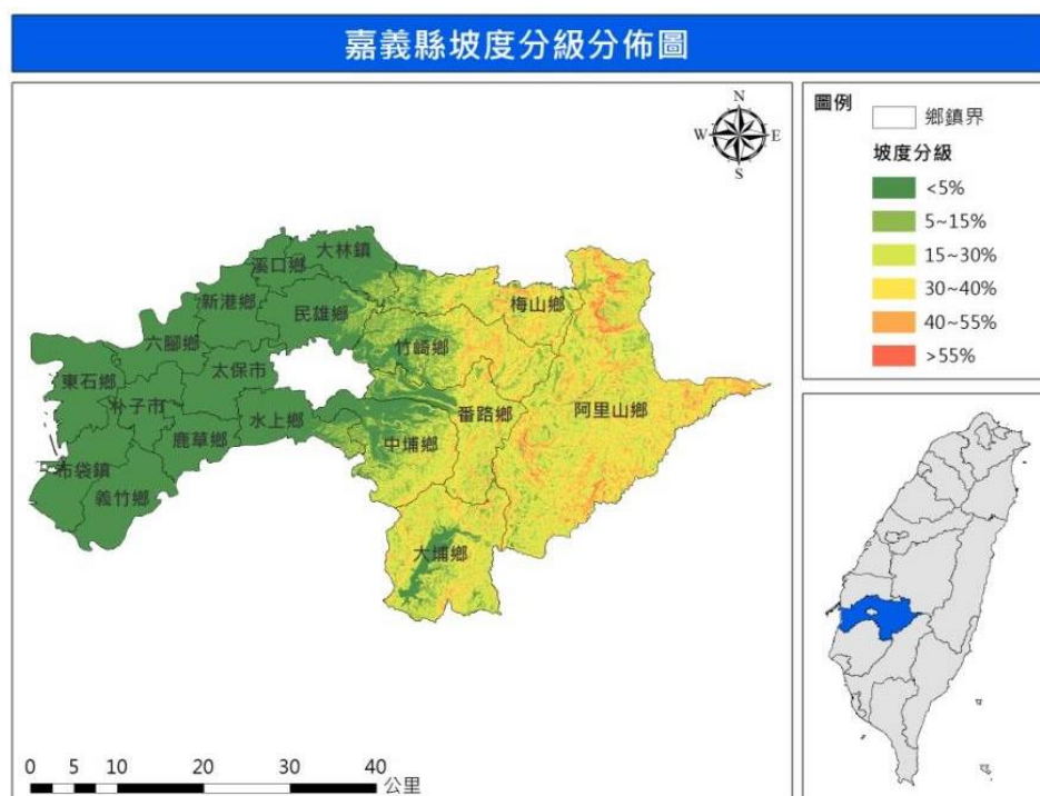
圖 1-2- 1 嘉義縣坡地分級分佈圖
