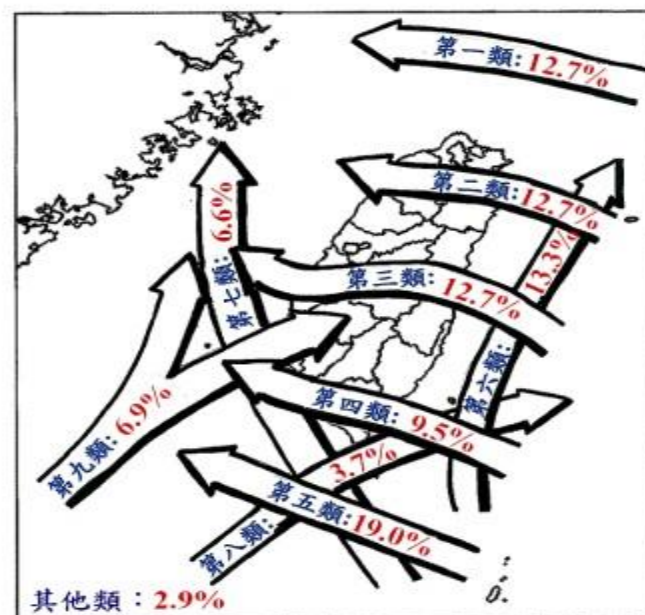
圖 2-1- 1 影響臺灣地區颱風路徑分類圖(1911—2010 年)
