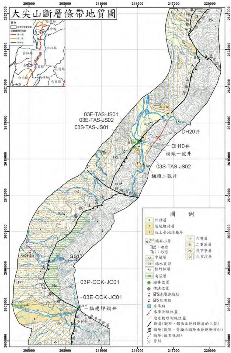
圖 1-2- 12 大尖山斷層地質圖。圖中顯示地球物理測線與鑽探位置。(坐標系統：
