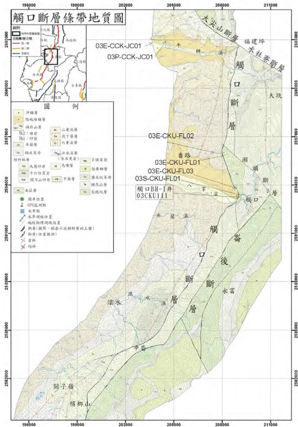
圖 1-2-9 觸口斷層地質圖。圖中指示鑽井位置與地球物理測線。(坐標系統：TWD67)
