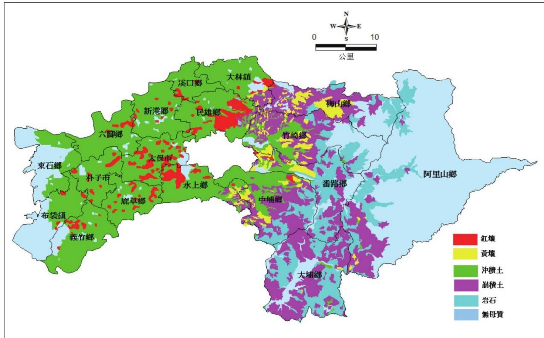
圖 1-2-2 嘉義縣地質分布圖
