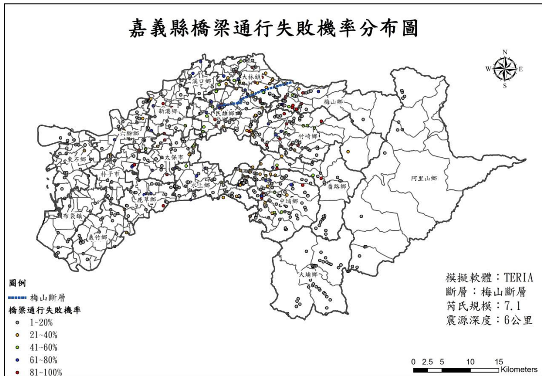
圖 3-2-12 嘉義縣橋樑通行失敗機率分布圖
