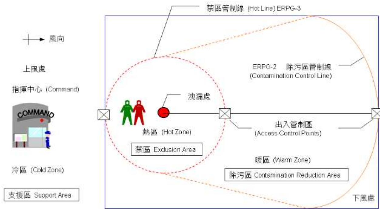
圖四、毒性及關注化學物質災害管制區域劃分示意圖
