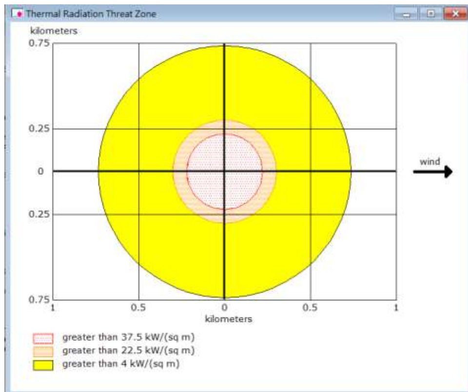
圖 15-8 二甲苯池火模式熱輻射影響範圍
