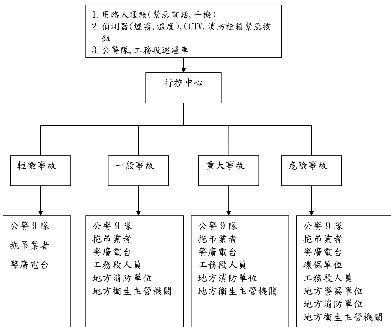
圖 7-9 雪山隧道緊急事故通報流程圖
