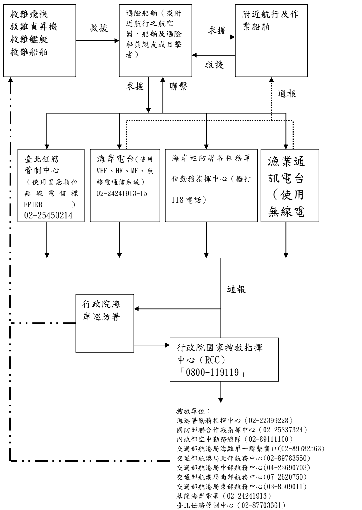
圖 14-2 海難遇險警報及訊息之接收與流程
