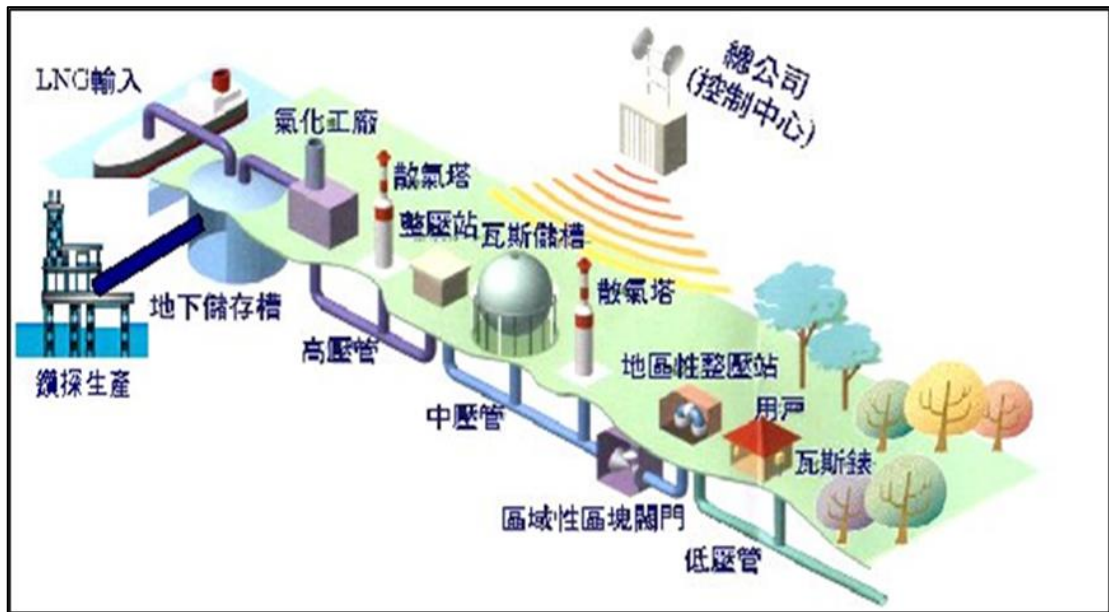
圖3-20 瓦斯系統配置示意圖
