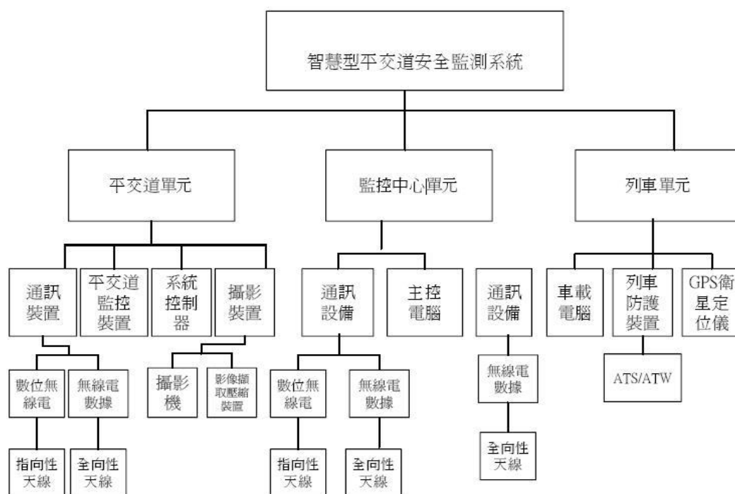
圖 8-8 平交道安全監測系統架構
