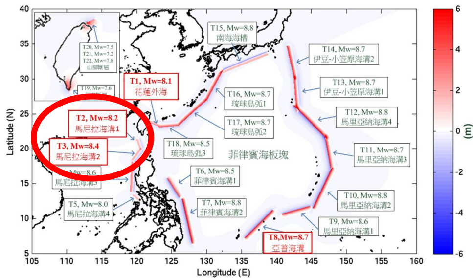
圖 4-5 台灣外海易形成海嘯之斷層分布圖(如紅圈處)
