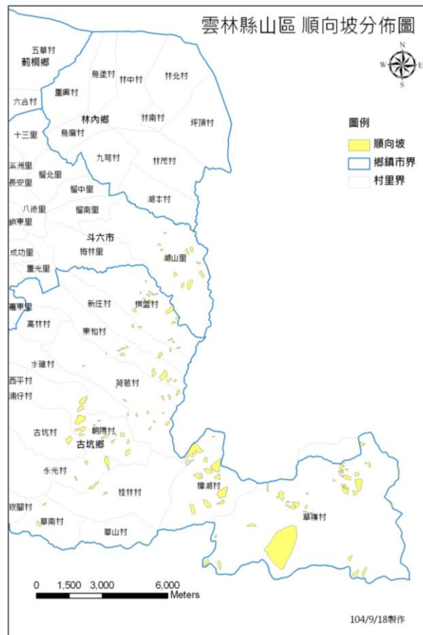
圖 3-22 雲林縣山區順向坡分佈圖
