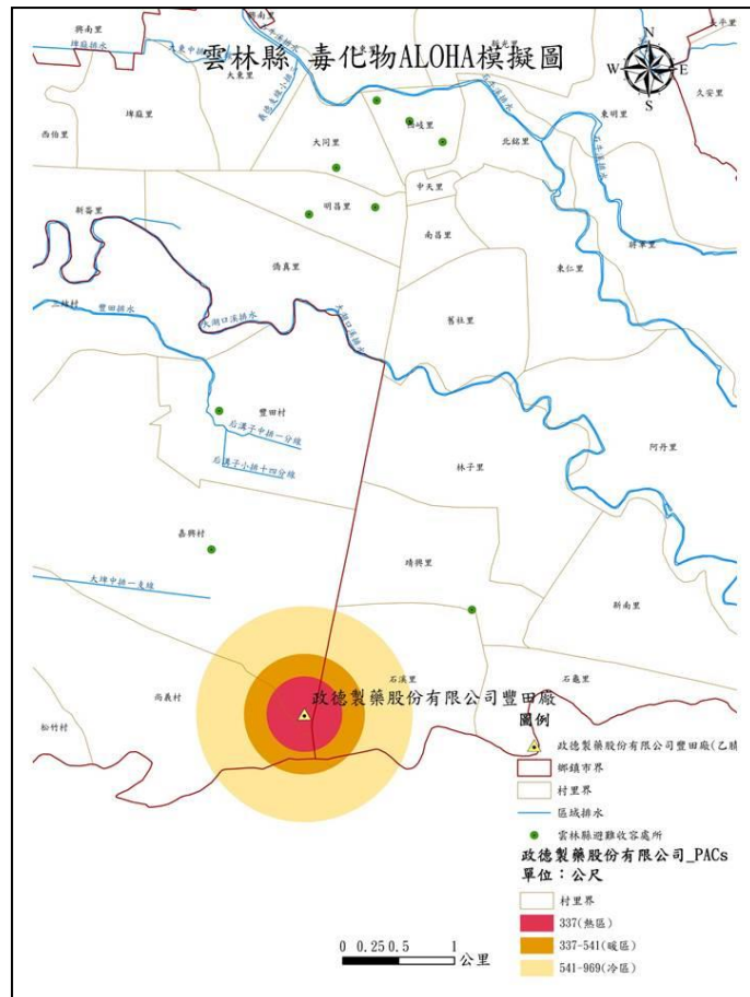
圖 6-2 豐田工業區毒化災模擬圖
