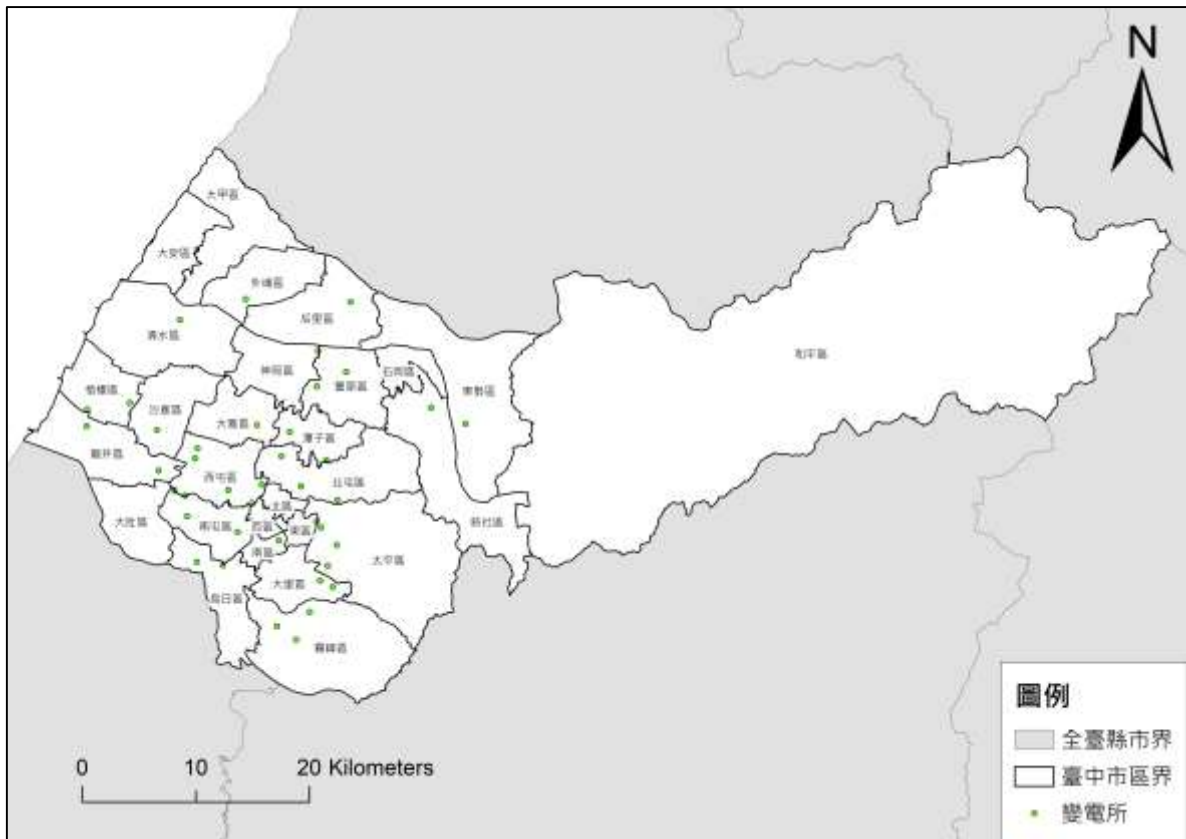
圖 1-3-87 臺中市變電所位置分布圖
