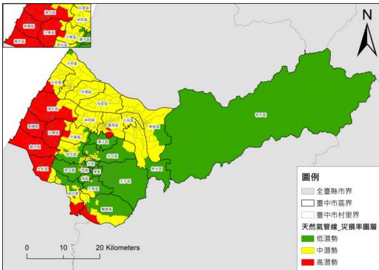
圖 1-3-92 臺中市天然氣管線災損率分布圖
