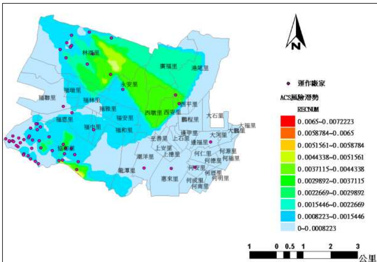
圖 1-3-67 臺中市西屯區一般洩漏模擬情境(ACS)毒性化學物質危害風險潛勢圖(範例)
