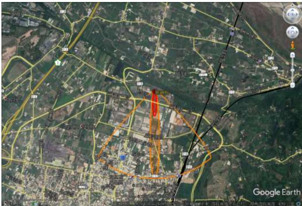
圖 1-3-63 臥式氯氣鋼瓶 ALOHA 一般洩漏情境影響範圍
