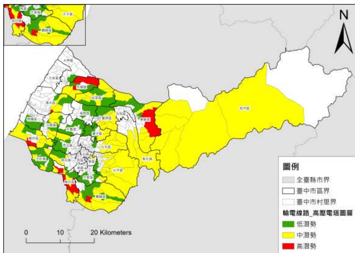
圖 1-3-110 臺中市各里高壓電塔分布圖
