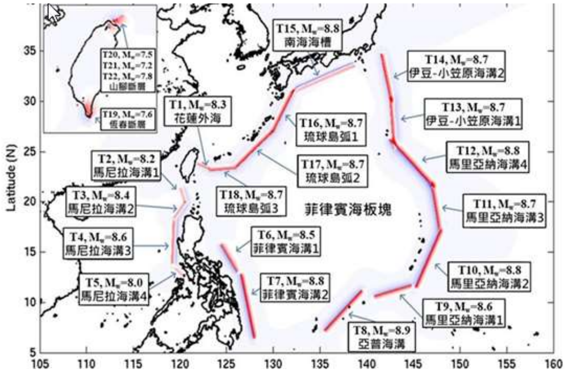
圖 1-3-54 海溝型海嘯源編號、地震矩規模與分布位置圖
