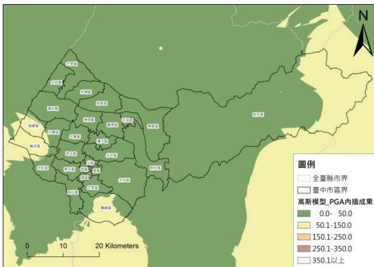
圖 1-3-91 高斯模型 PGA 資料內插成果圖
