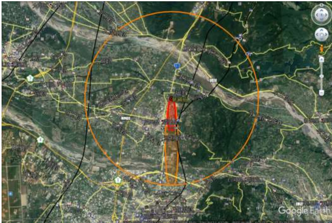
圖 1-3-62 臥式氯鋼瓶 ALOHA 最嚴重模擬情境影響範圍
