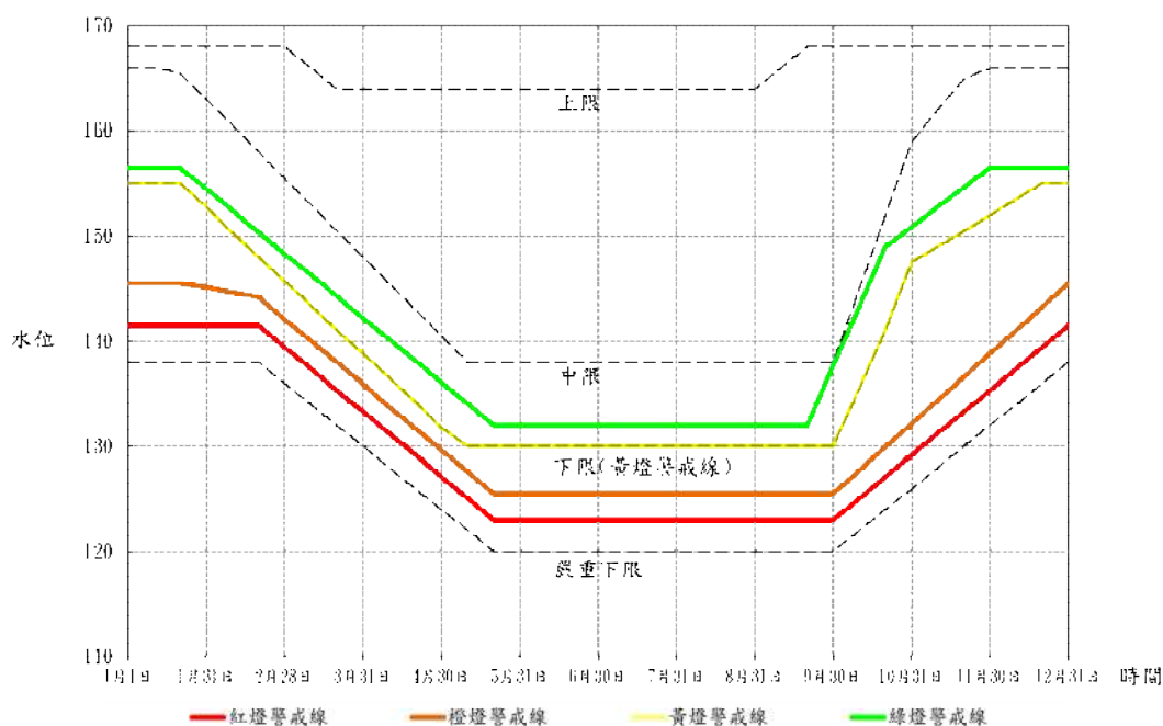
圖 1-3-5-3 翡翠水庫燈號警戒線示意圖
