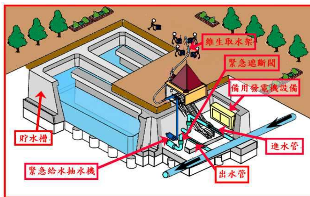
圖 4-3-1-3 鋼筋混凝土維生貯水槽之加壓站配水池示意圖
