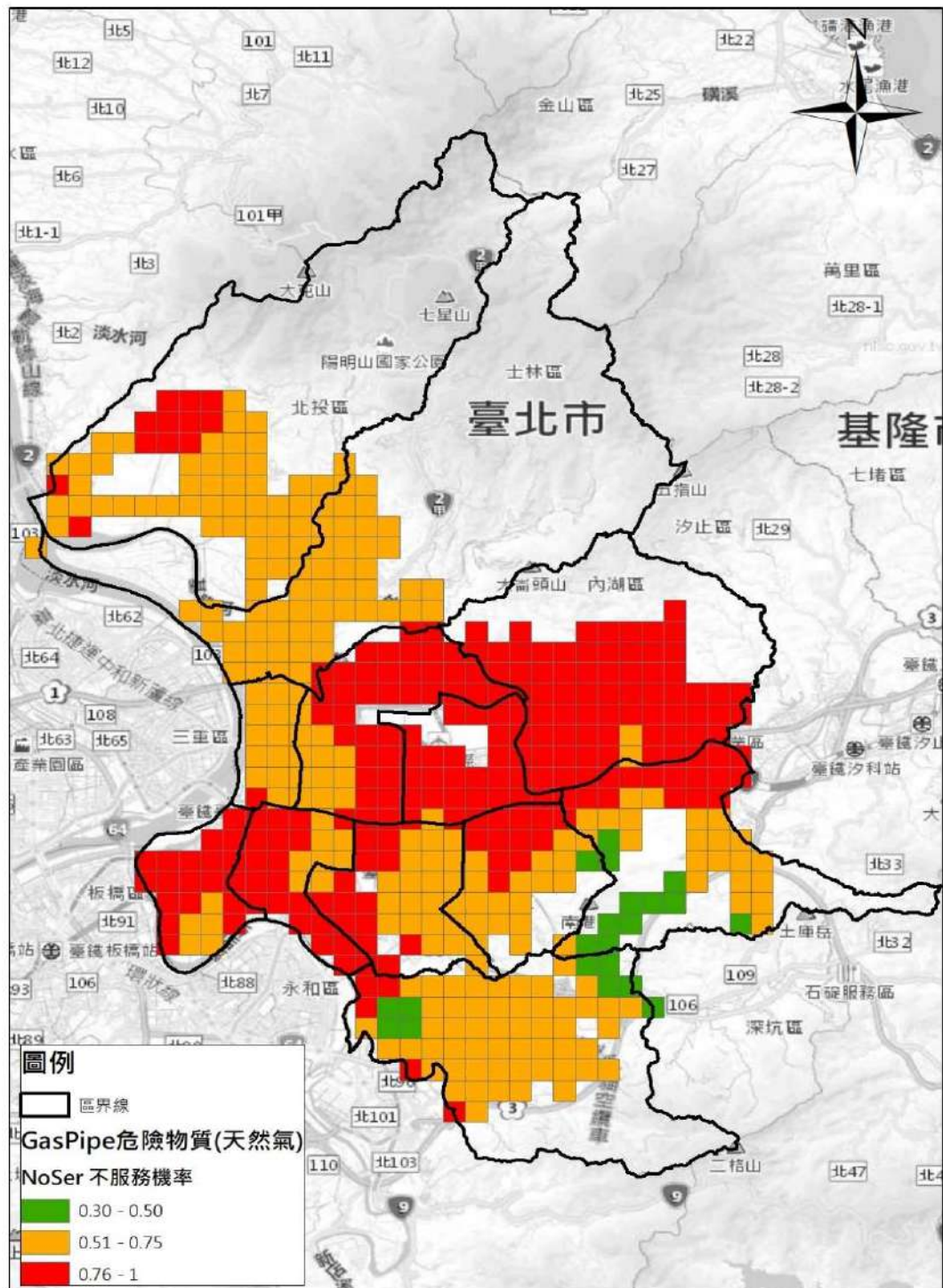
圖 1-3-3-10 TERIA 系統模擬-天然氣不服務機率分布圖
