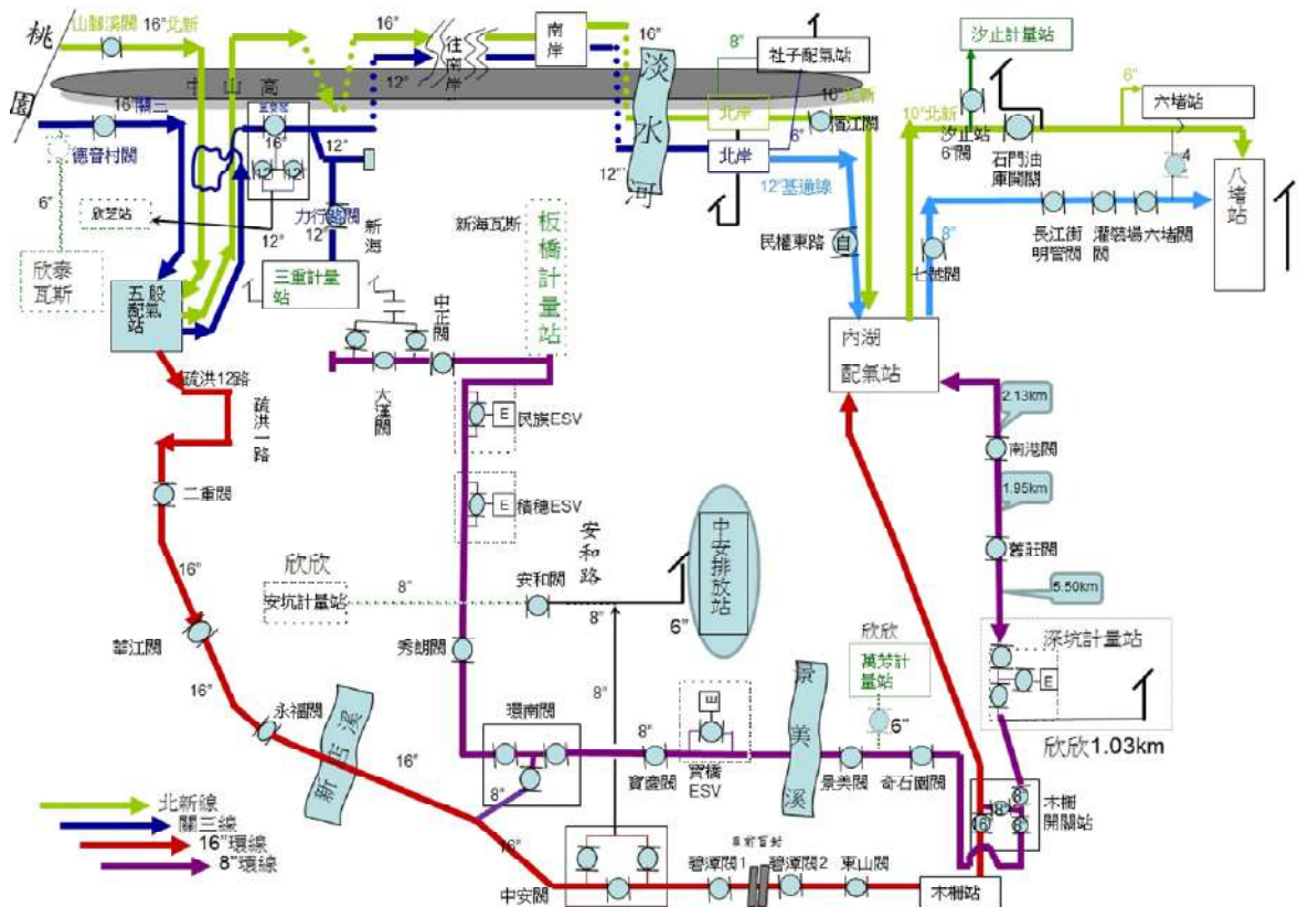
圖 1-3-9-2 臺灣中油公司天然氣輸送系統圖
