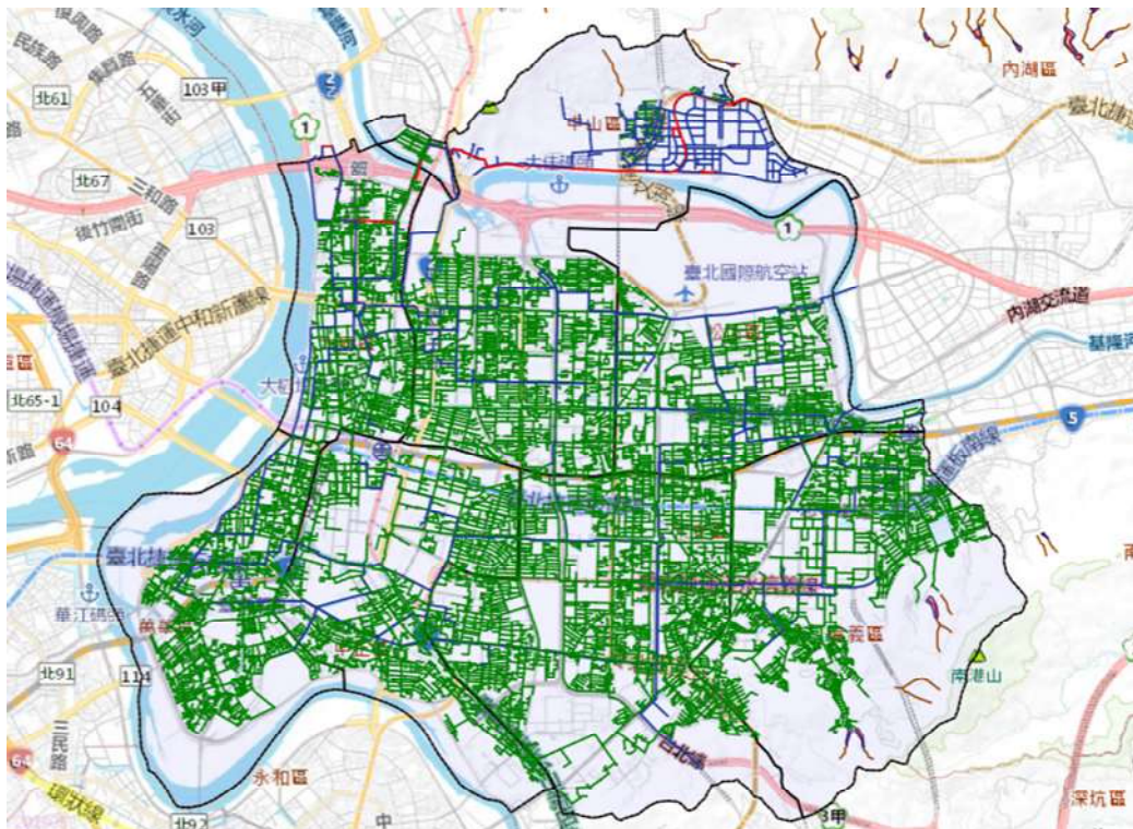
圖 4-3-12-1 大台北區瓦斯股份有限公司管線套繪圖
