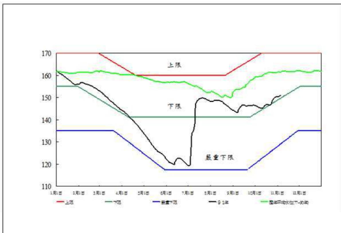
圖 1-3-5-1 91 年翡翠水庫水位歷線圖
