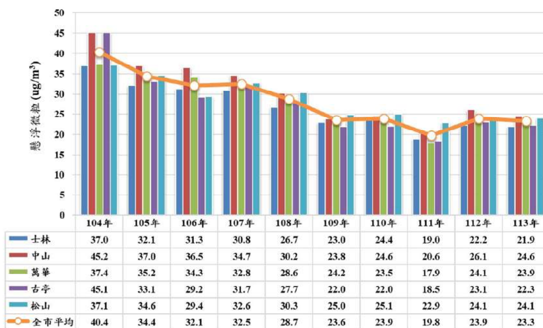
圖 1-3-20-1 環境部監測站近 10 年 PM 10 年平均濃度變動趨勢
