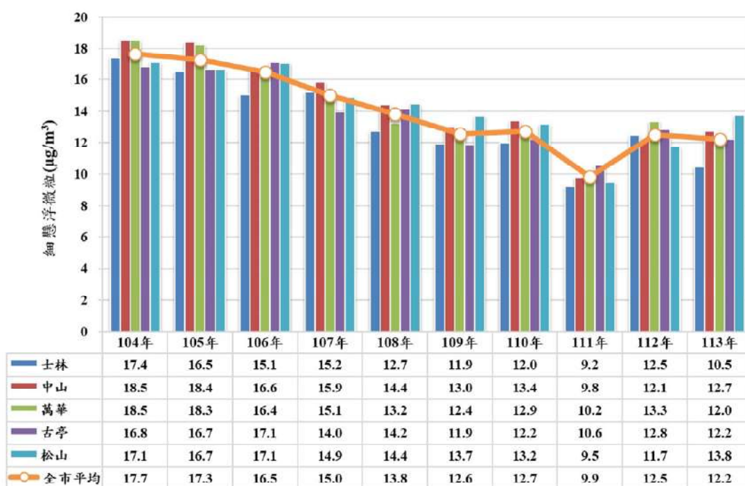
圖 1-3-20-2 環境部監測站近 10 年 PM 2.5 年平均濃度變動趨勢
