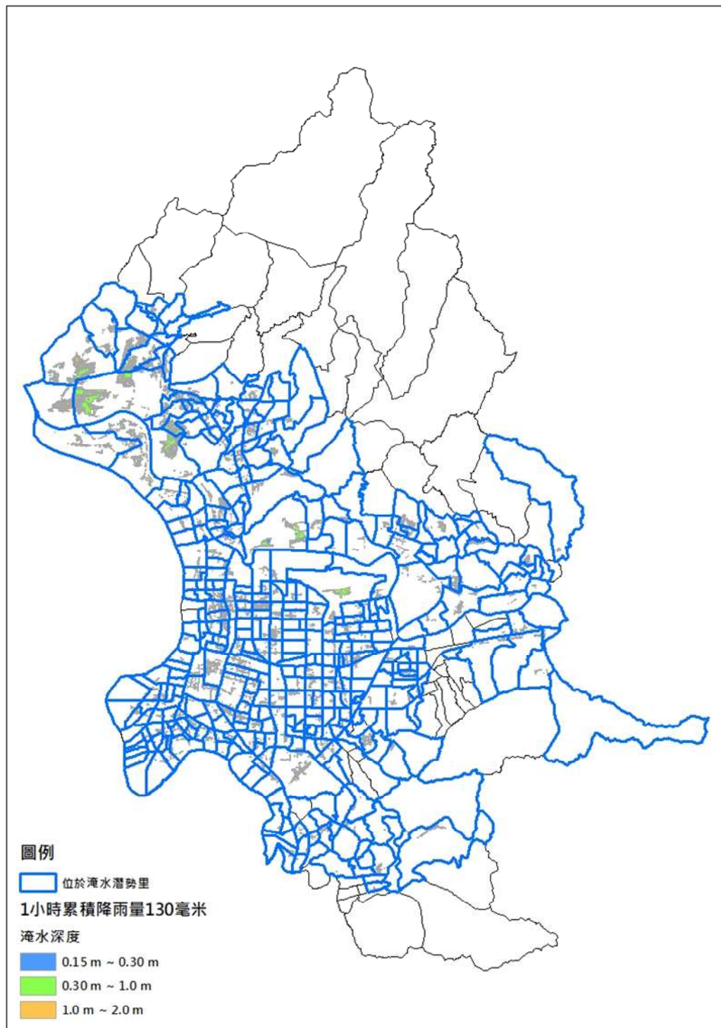
圖 1-4-2-4 臺北市政府工務局水利工程處短延時強降雨 淹水模擬 1 小時降雨 130 毫米
