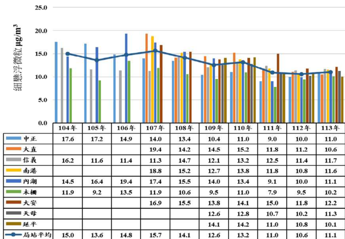
圖 1-3-20-4 臺北市環保局監測站近 10 年 PM 2.5 年平均濃度變動趨勢
