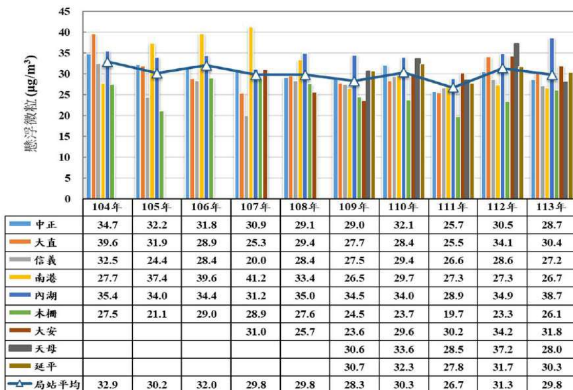
圖 1-3-20-3 臺北市環保局監測站近 10 年 PM 10 年平均濃度變動趨勢
