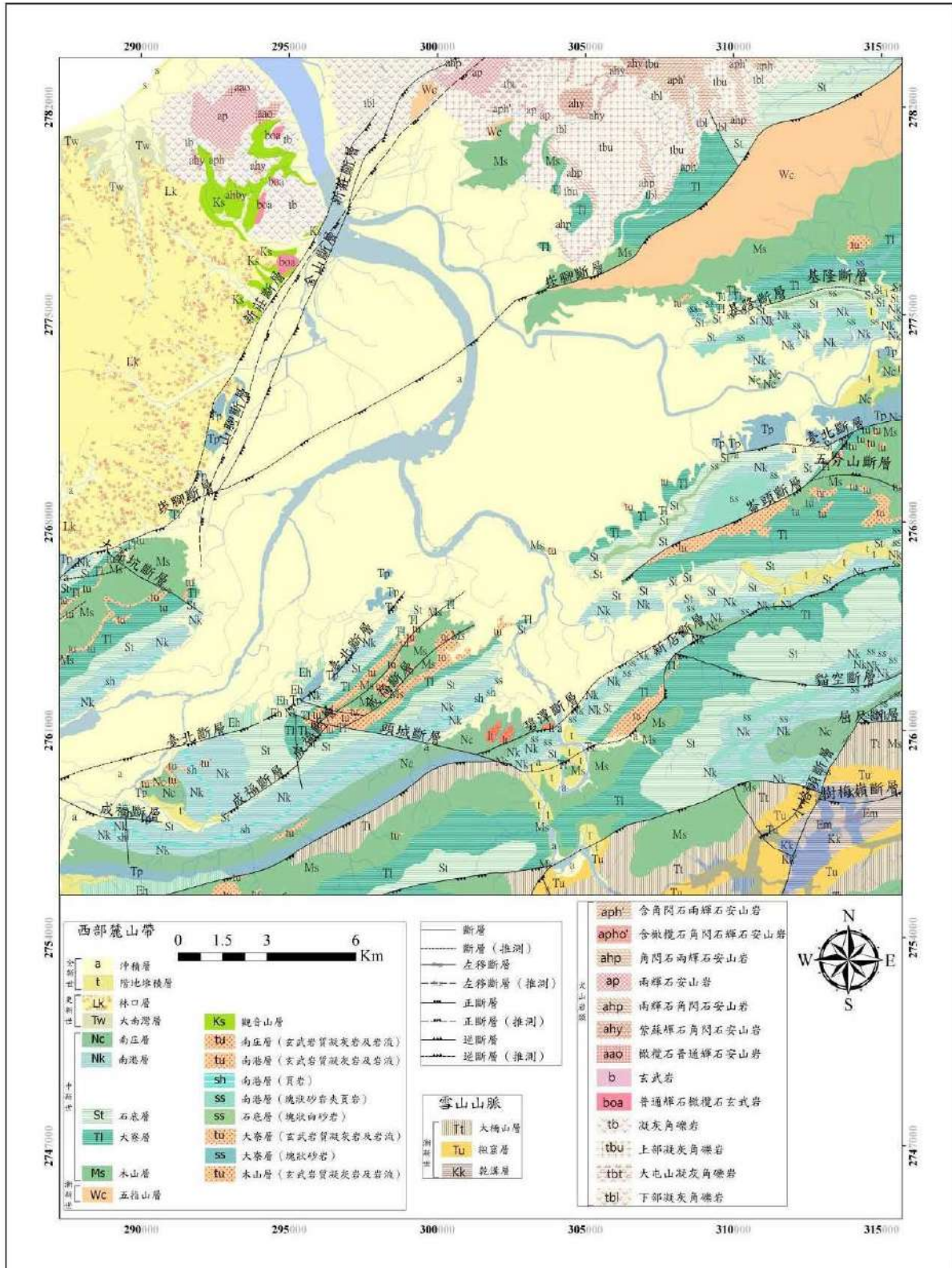
圖 1-2-2-2 地質圖
