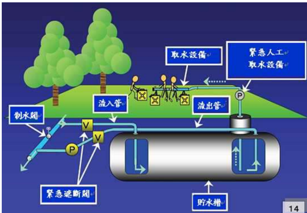
圖 4-3-1-2 管狀維生貯水槽示意圖
