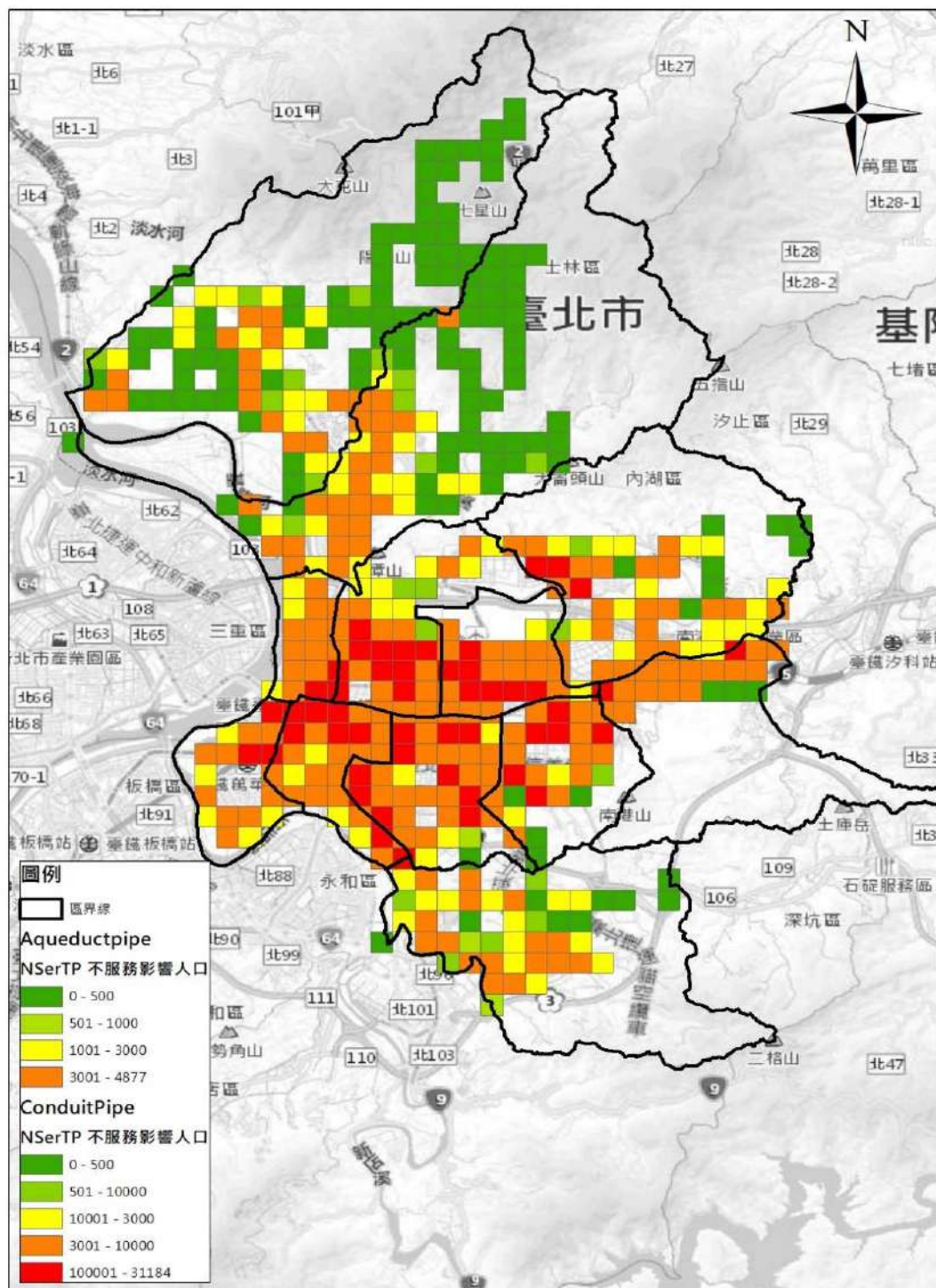
圖 1-3-3-11 TERIA 系統模擬-供水不服務影響人口分布圖
