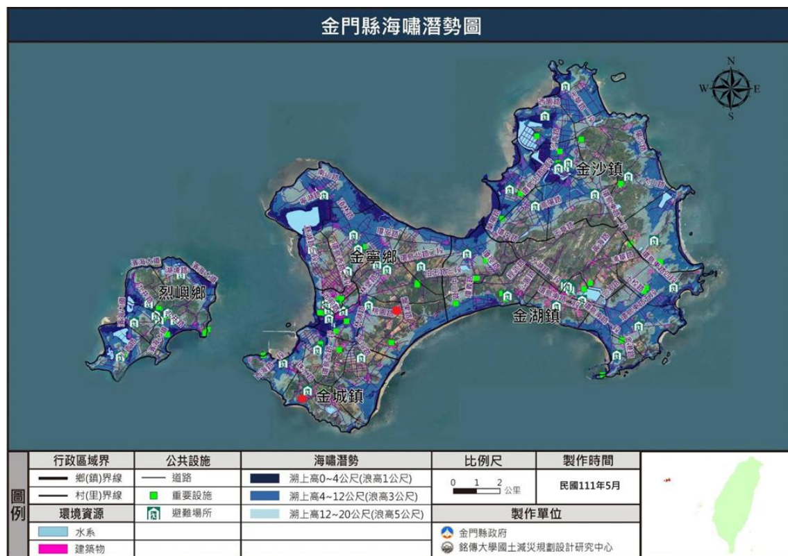
圖 26 金門縣海嘯潛勢圖
