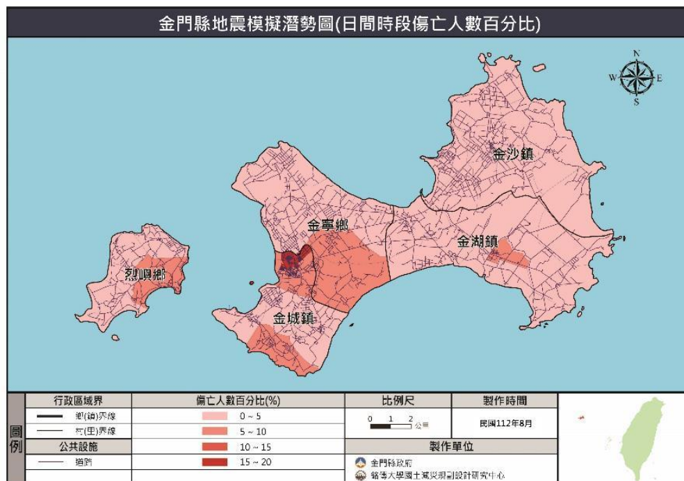
圖 20 金門縣地震模擬潛勢圖(日間時段傷亡人數百分比)
