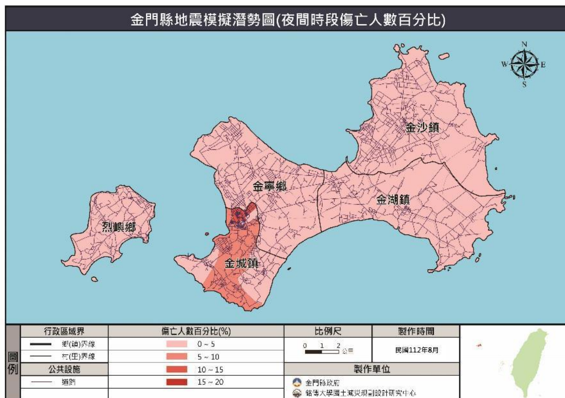
圖 21 金門縣地震模擬潛勢圖(夜間時段傷亡人數百分比)
