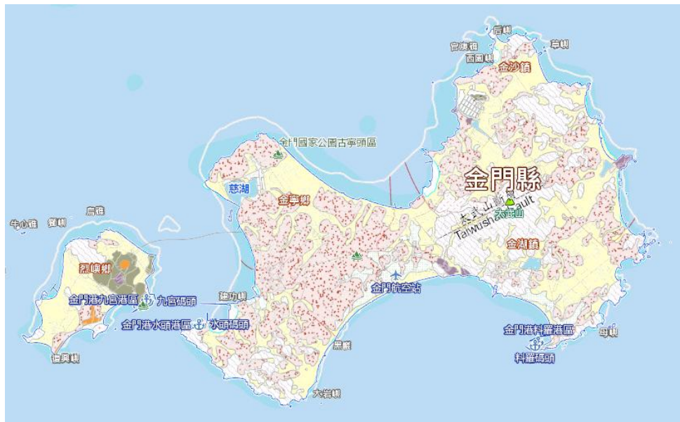
圖 3 金門地質圖
