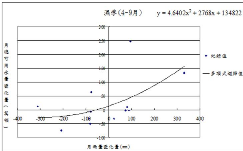
圖 16 濕季(4-9月)總可用水量與雨量變化迴歸分析圖
