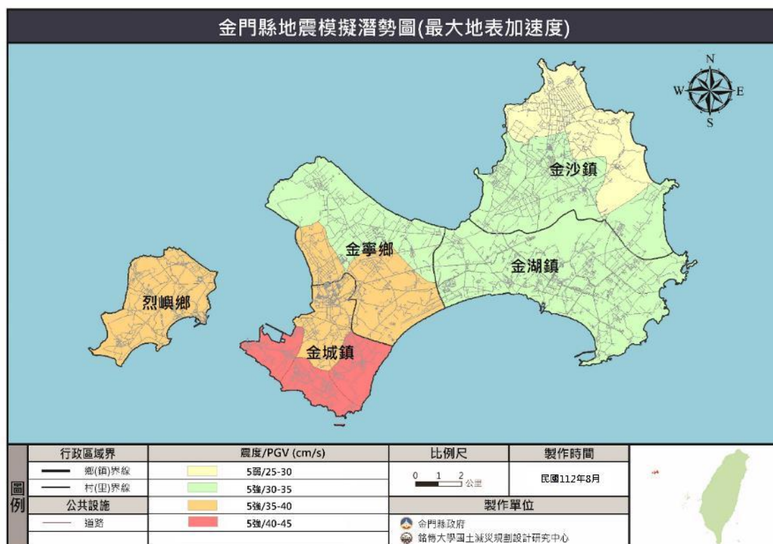
圖 24 金門縣地震模擬潛勢圖(最大地表加速度 PGA)
