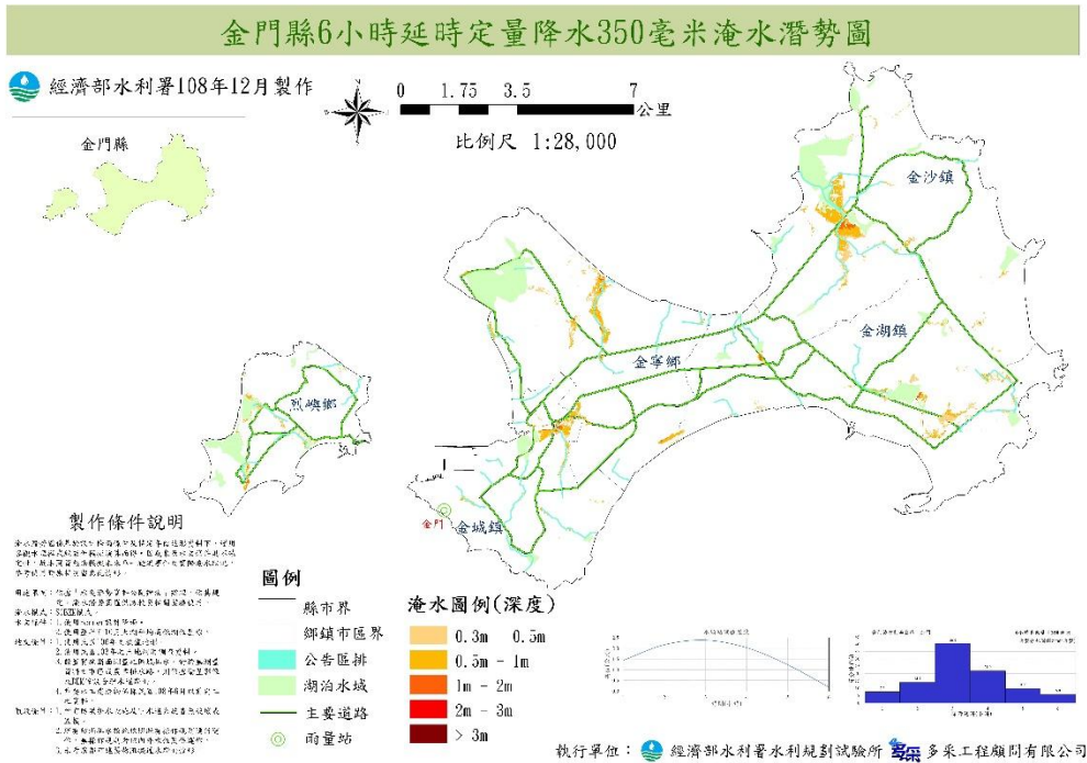
圖 13 金門縣 6 小時延時定量降水 350 毫米淹水潛勢圖
