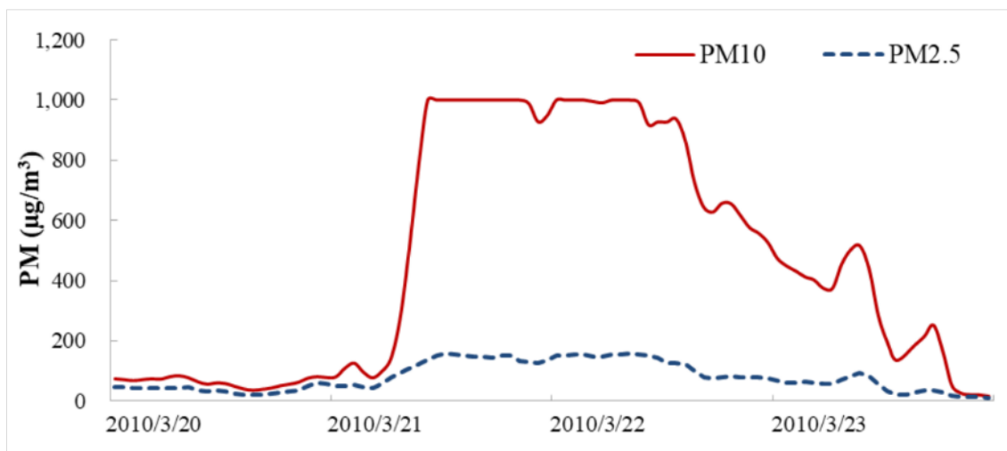
圖 28 本縣 2010 年 3 月 21~22 日 PM 10 及 PM 2.5 濃度變化
