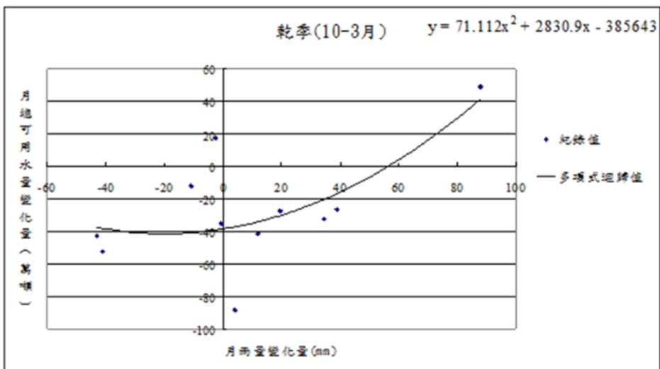
圖 17 乾季(10-3月)總可用水量與雨量變化迴歸分析圖
