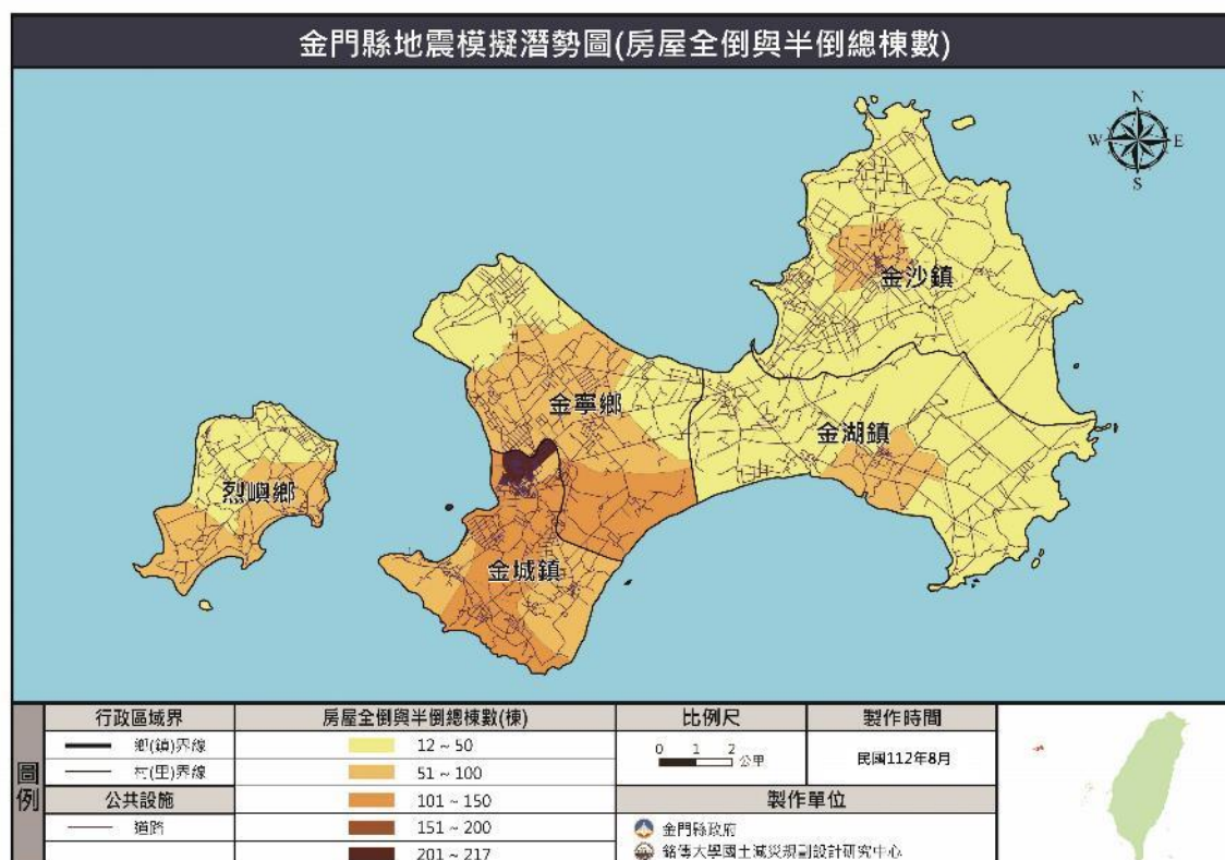
圖 22 金門縣地震模擬潛勢圖(房屋全倒與半倒總棟數)
