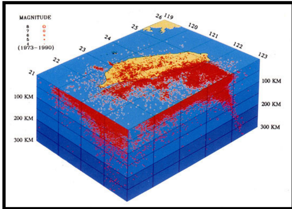
1-2-13 臺灣地震震源剖面圖(資料來源：中央大學工程地質研究室 2009)
