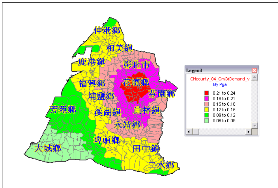
圖 3-1- 164 彰化斷層地震－地表震動強度 PGA 分佈
