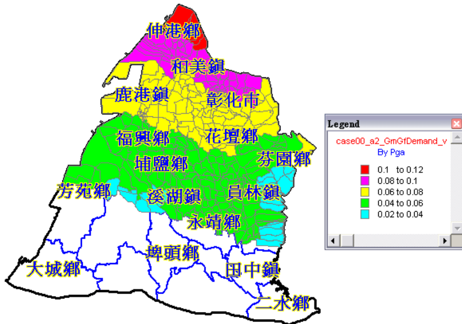
圖 3-1-3 地表震動強度 PGA 分布(事件二-大甲斷層地震)
