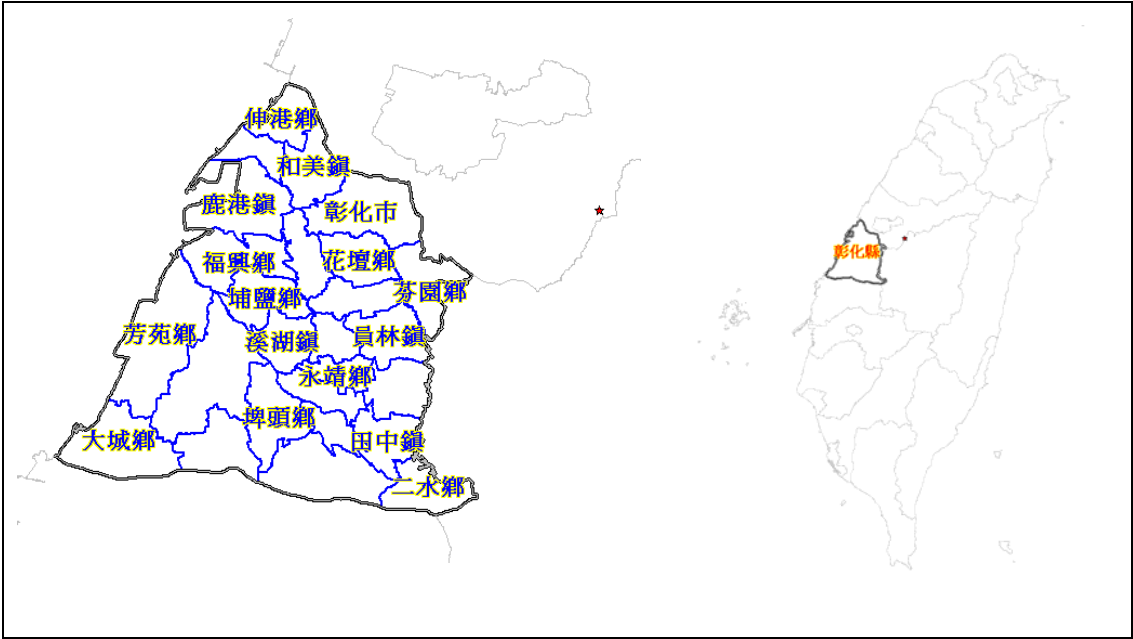
圖 3-1- 74 大茅埔-雙冬斷層地震－震央位置圖
