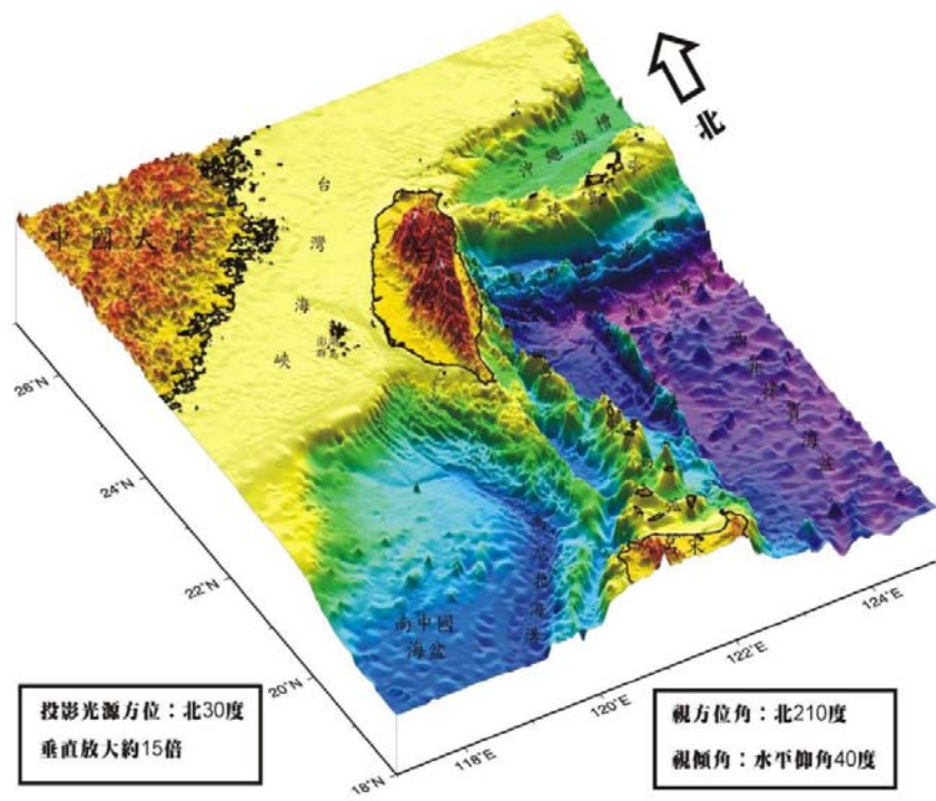
圖 9-5-2 馬尼拉海溝地體構造立體圖。(圖片來源：海科中心)
