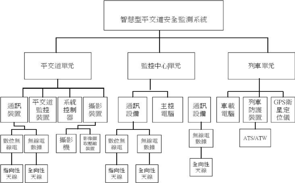
圖7-1-8平交道安全監測系統架構
