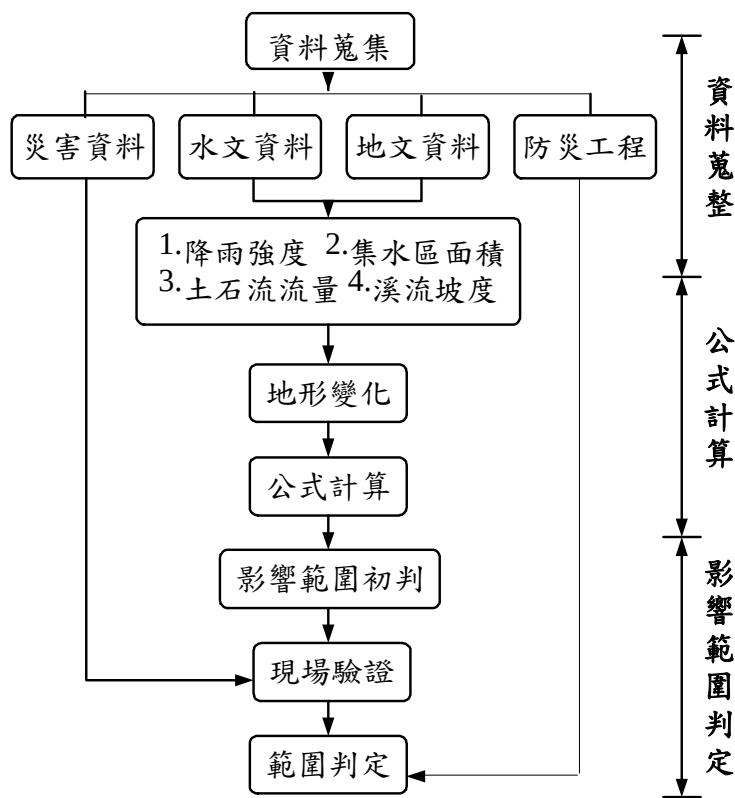
圖 4-1-5 土石流潛勢溪流潛勢判定流程
