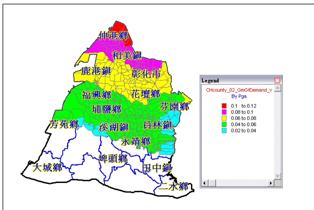
圖 3-1-16 事件二大甲斷層地震—地表震動強度 PGA 分佈
