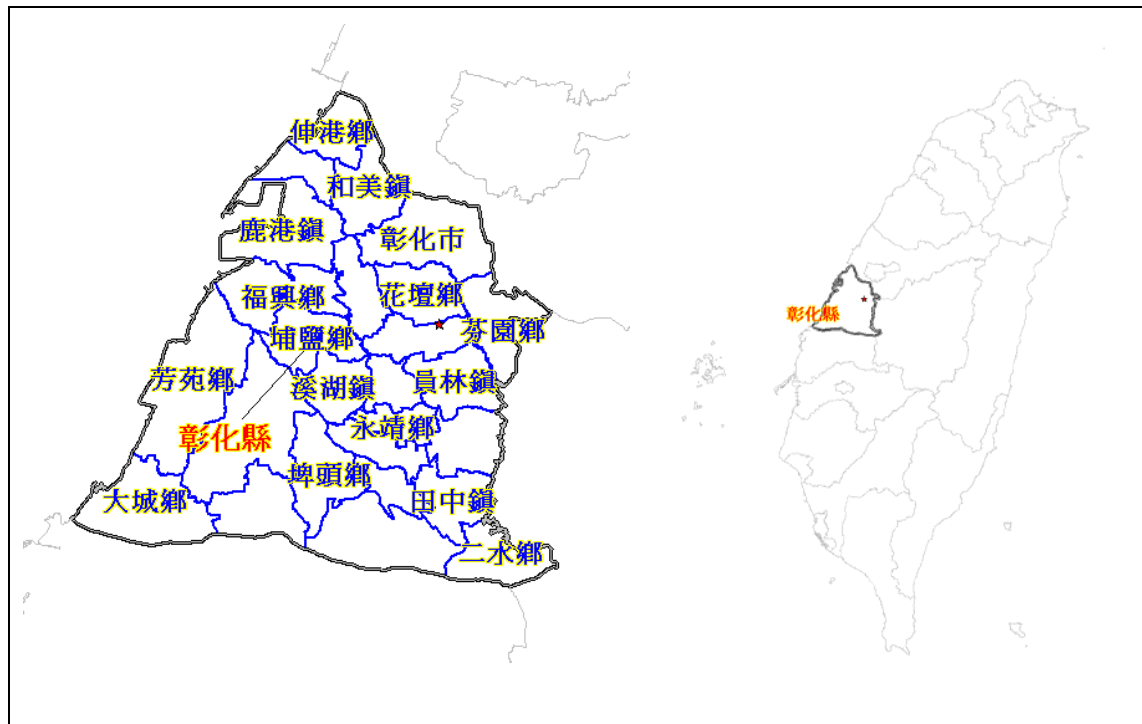
圖 3-1- 153 彰化斷層地震－震央位置圖
