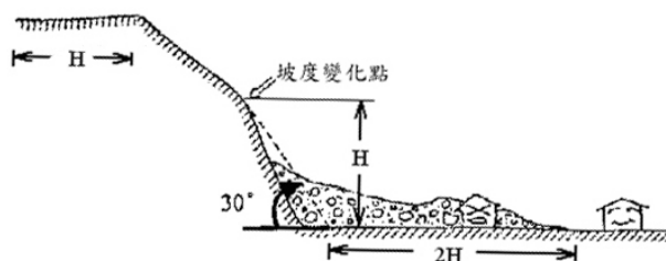
圖 4-1-8 崩塌地示意圖
